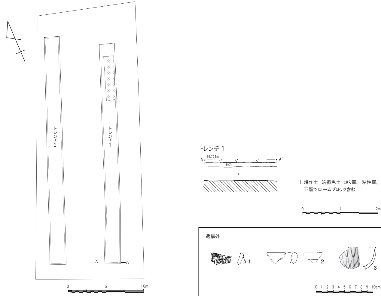
第 5 図 北野遺跡第 51 地点調査区域図 (1/300)、土層 (1/60)、出土遺物 (1/4)
