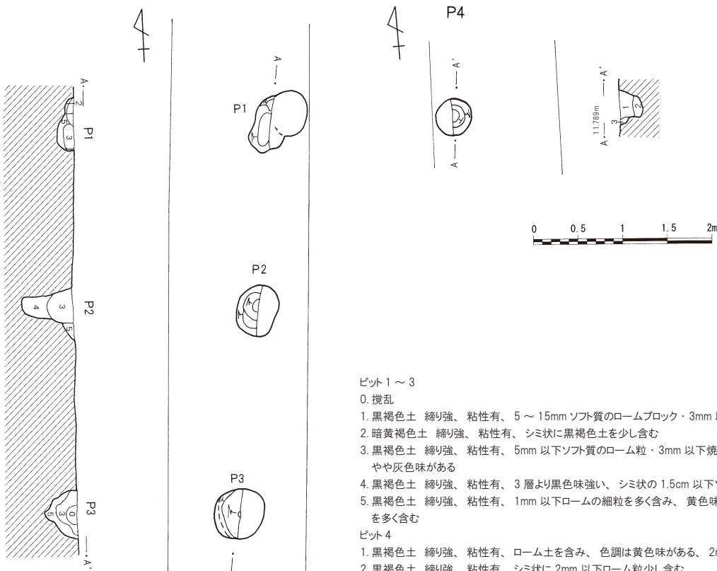
第15図 川崎遺跡第36地点ピット(1/60)
