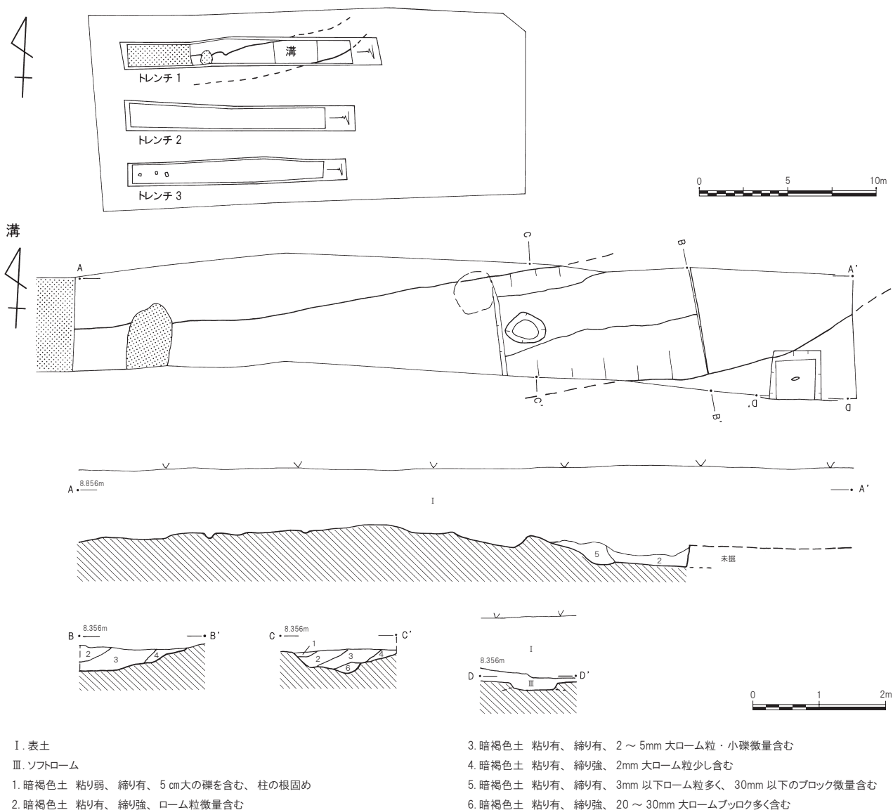
第 11 図 川崎遺跡第 45 地点遺構配置図 (1/300)、溝 (1/80)
