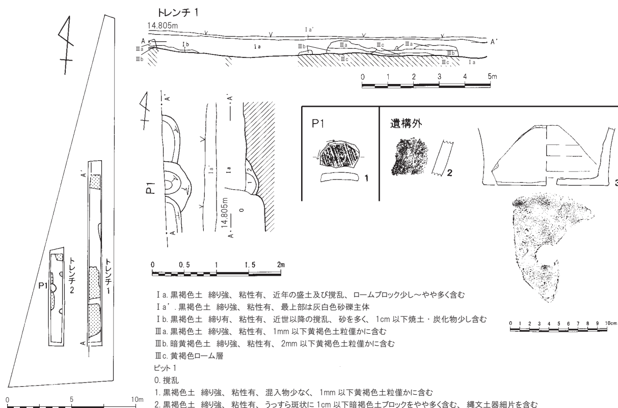
第9図 ハケ遺跡第12地点遺構配置図(1/300)、土層(1/150)、ピット(1/60)、出土遺物(1/4)
