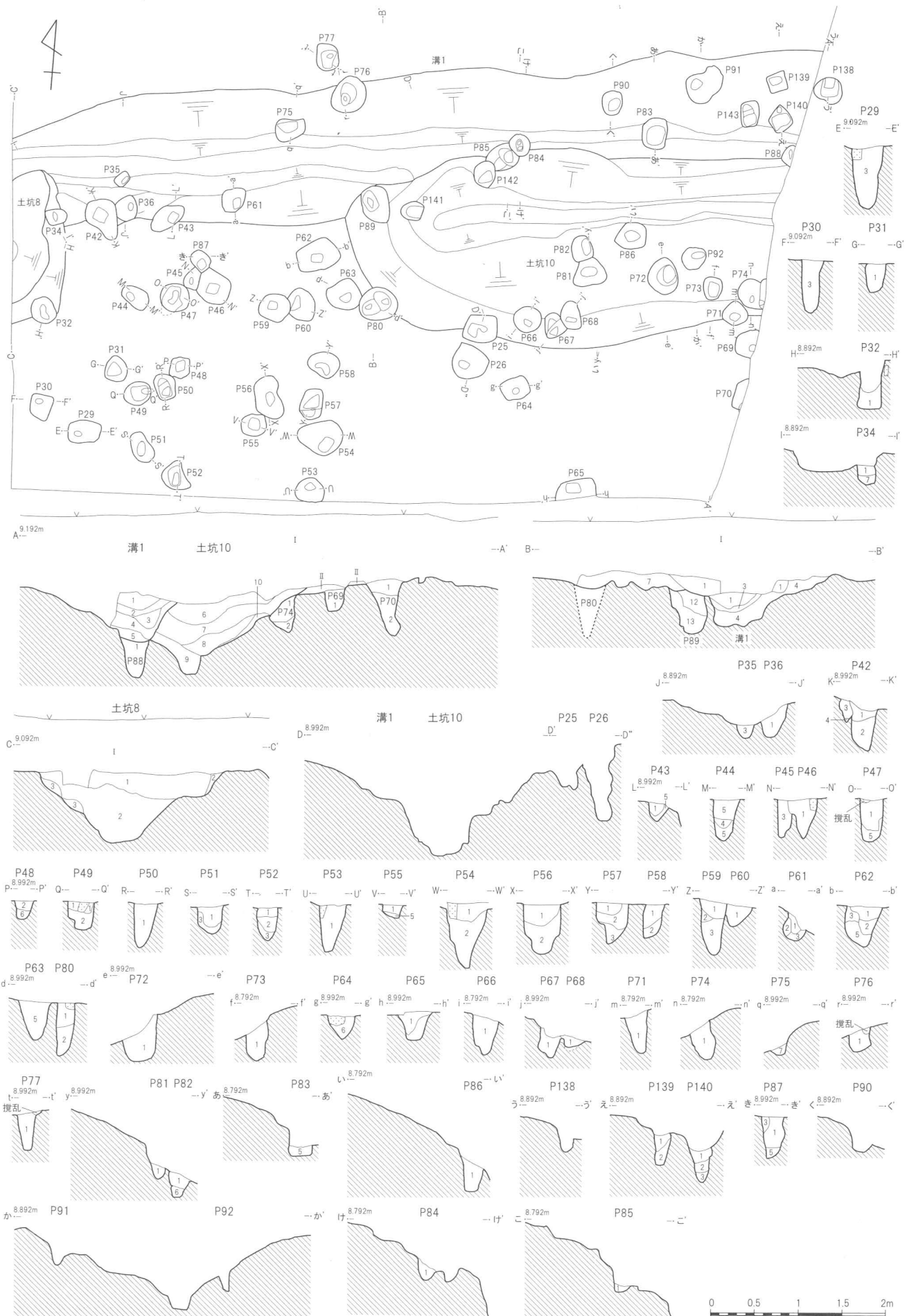
第19図 長宮遺跡第32地点土坑①・ピット①・溝① (1/60)
