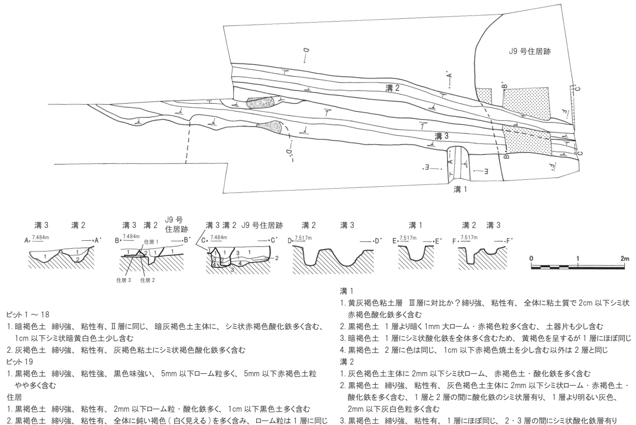
第 13 図 長宮遺跡第 34 地点溝 (1/80)
