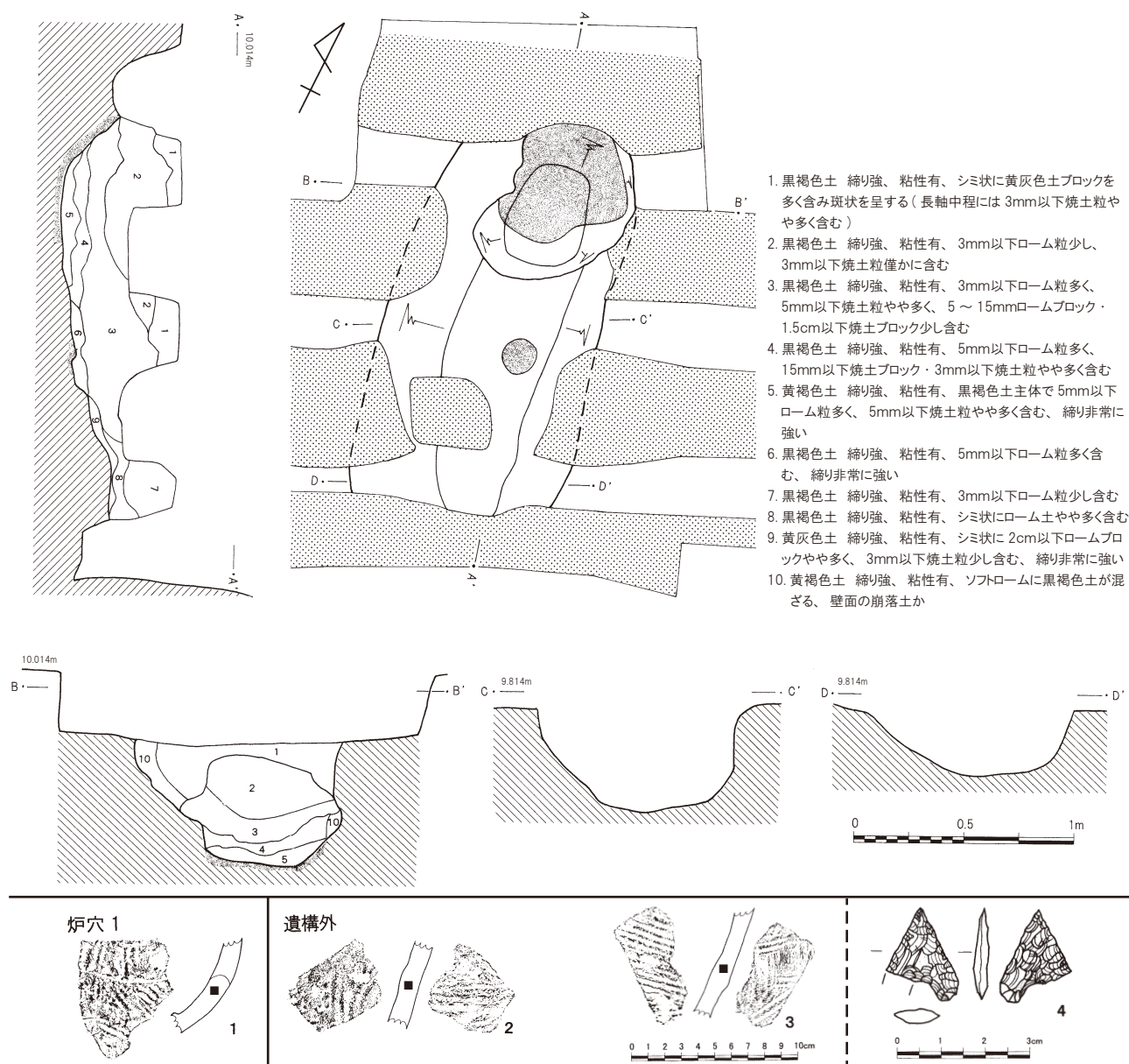
第 38 図 長宮遺跡第 35 地点炉穴 (1/30)、出土遺物 (1/4・2/3)
