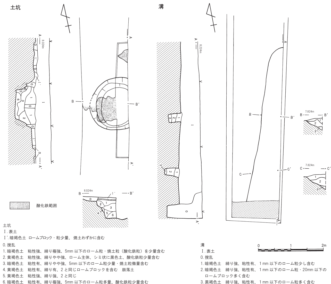
第 53 図 長宮遺跡第 54 地点土坑・溝 (1/60)
