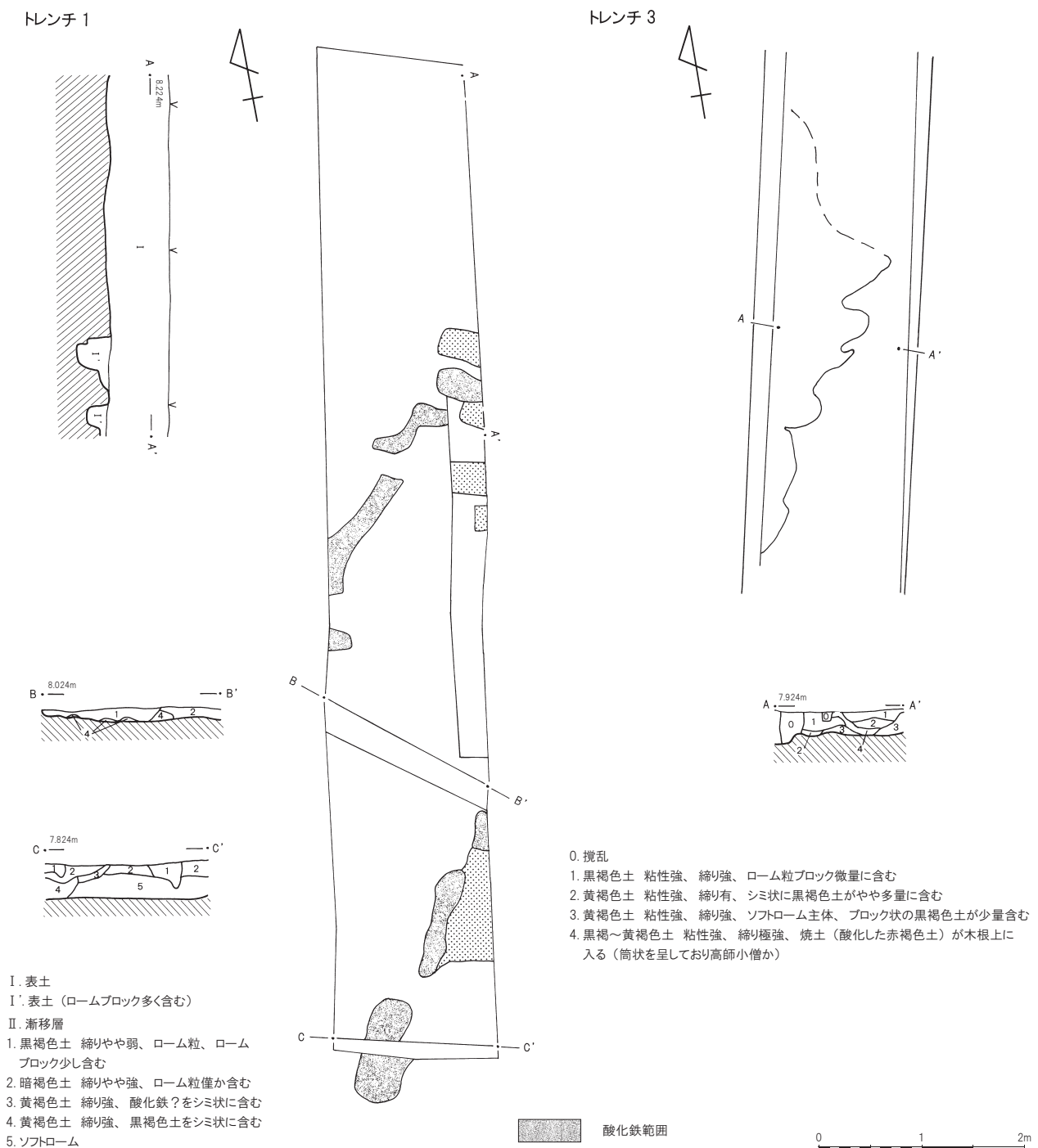
第 52 図 長宮遺跡第 54 地点トレンチ 1・3 酸化鉄範囲 (1/60)
