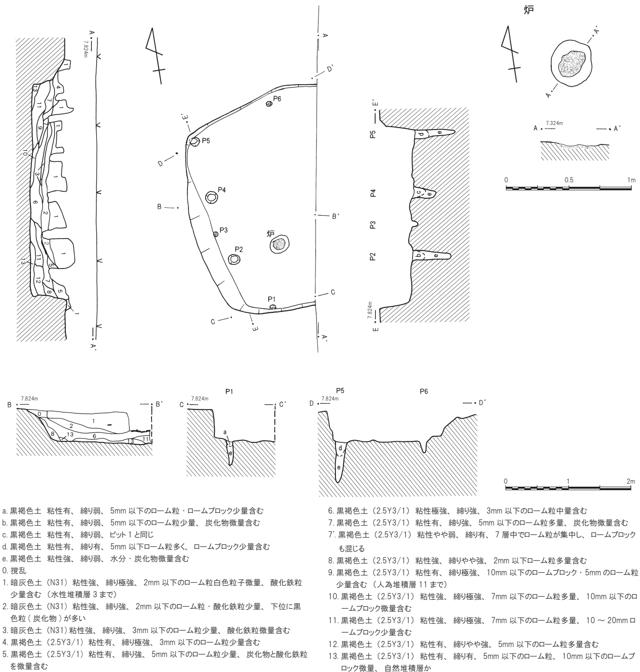
第50図 長宮遺跡第54地点J18号住居跡 (1/60)、炉 (1/30)
