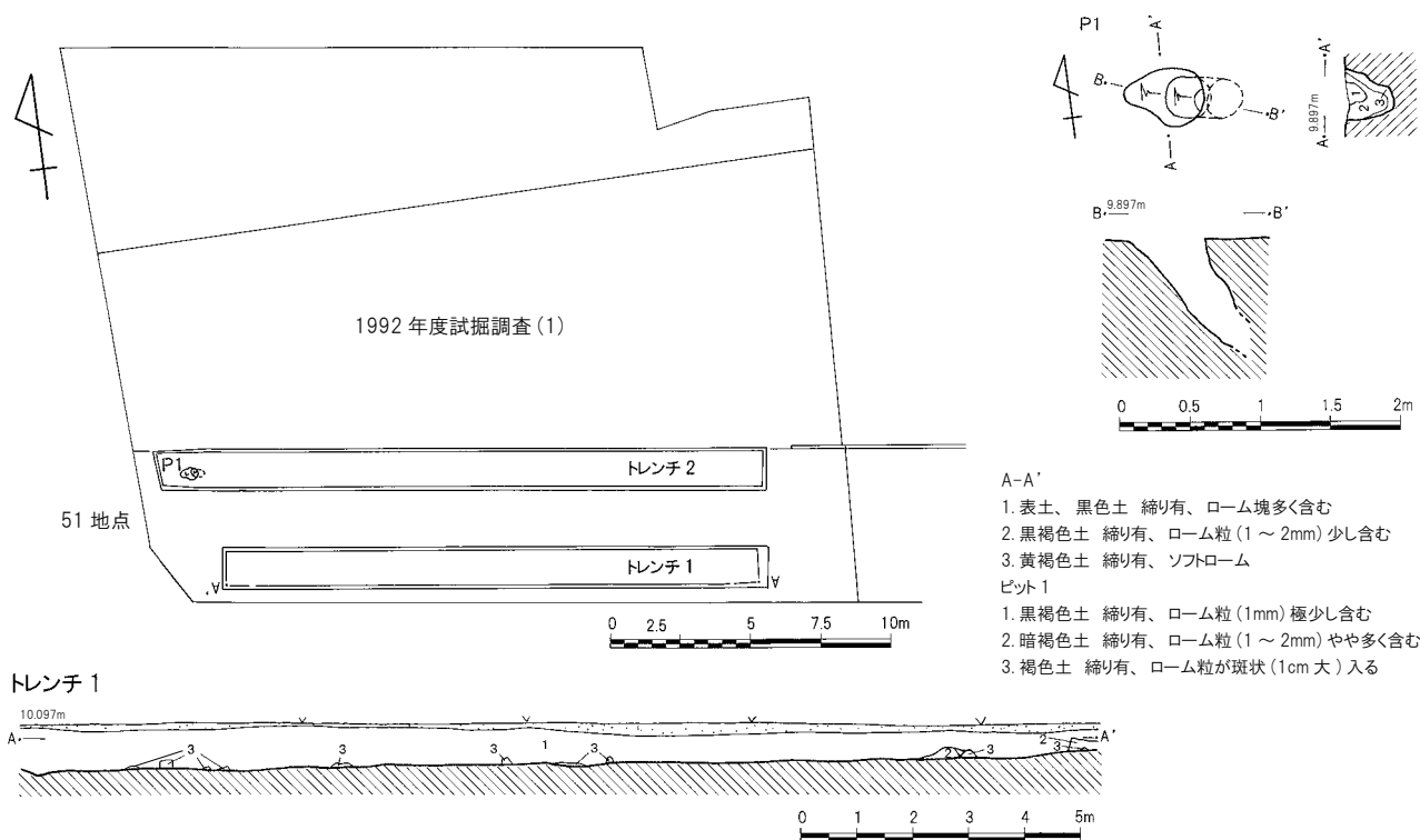
第 27 図 松山遺跡第 51 地点遺構配置図 (1/300)、土層図 (1/150)、ピット (1/60)
