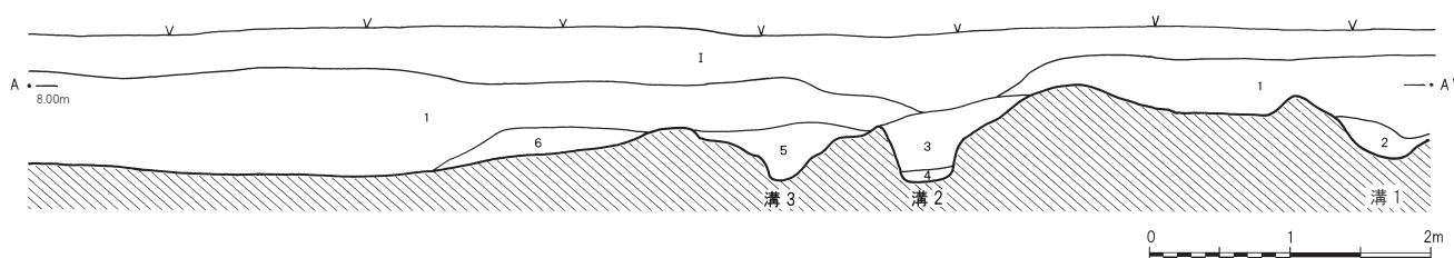
第73図 松山遺跡第90地点調査区域図・第91地点遺構配置図(1/300)、土層(1/60)、出土遺物(1/4・1/1)
