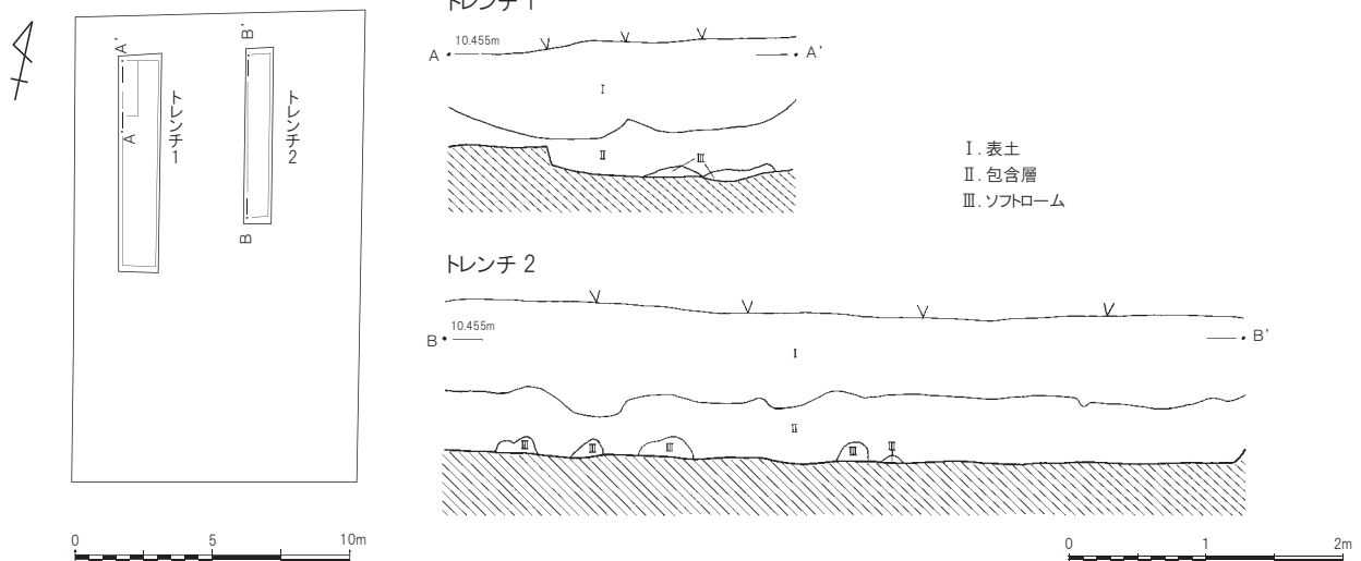
第22図 松山遺跡第112・113地点調査区域図(1/300)、土層(1/60)、出土遺物(1/4)
