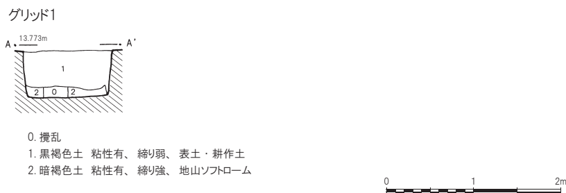
第 27 図 駒林遺跡第 43 地点遺構配置図・第 44 地点調査区域図 (1/300)、土層 (1/60)
