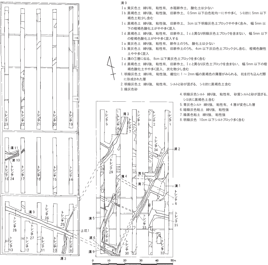
第 56 図 伊佐島遺跡第 4 地点遺構配置図 (1/1,000)
