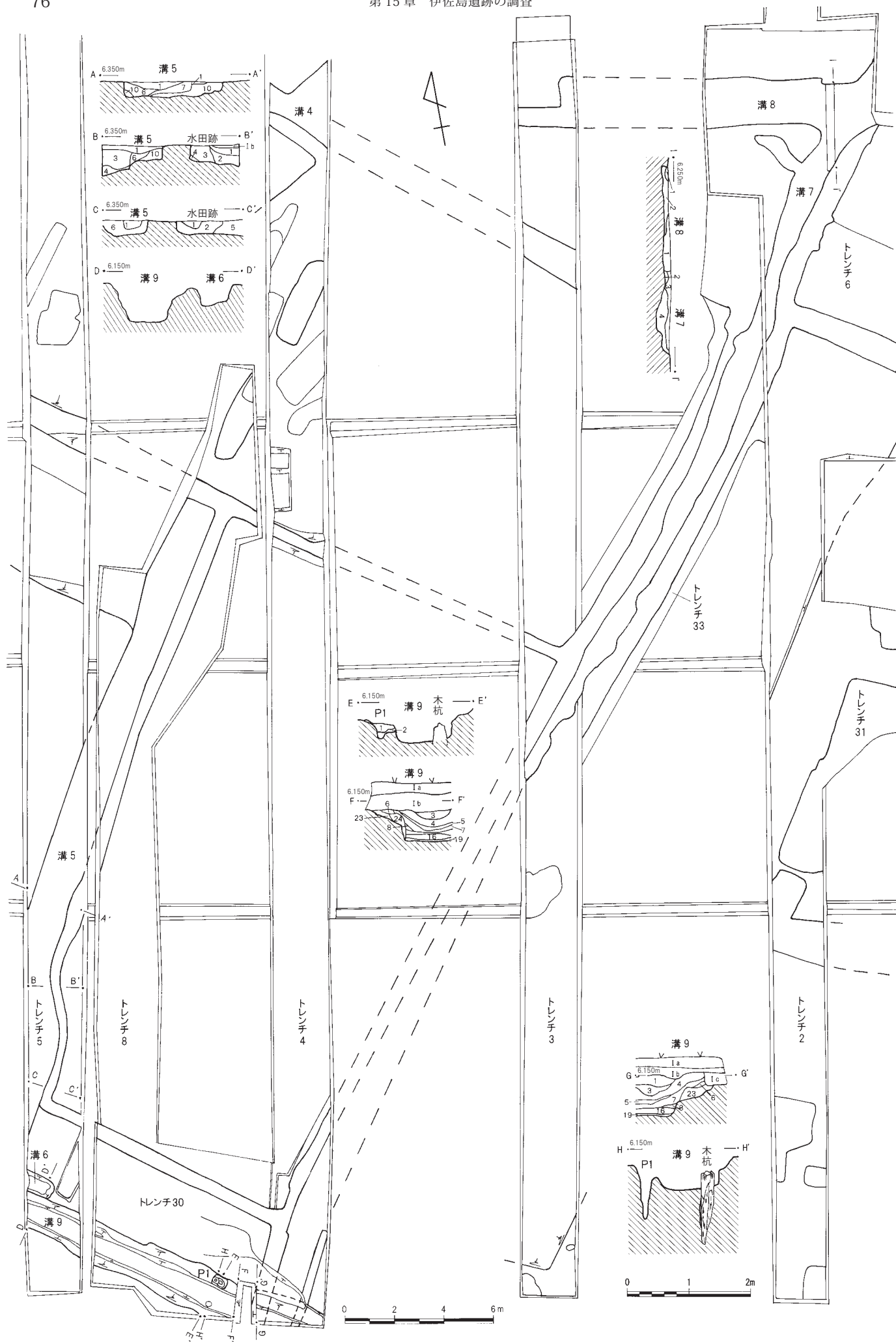
第58図 伊佐島遺跡第4地点ピット・溝② (1/200)、土層 (1/80)
