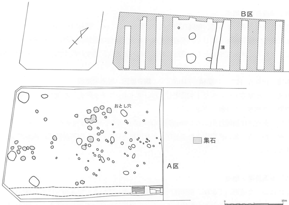
亀居遺跡第38地点遺構配置図(1/800)
