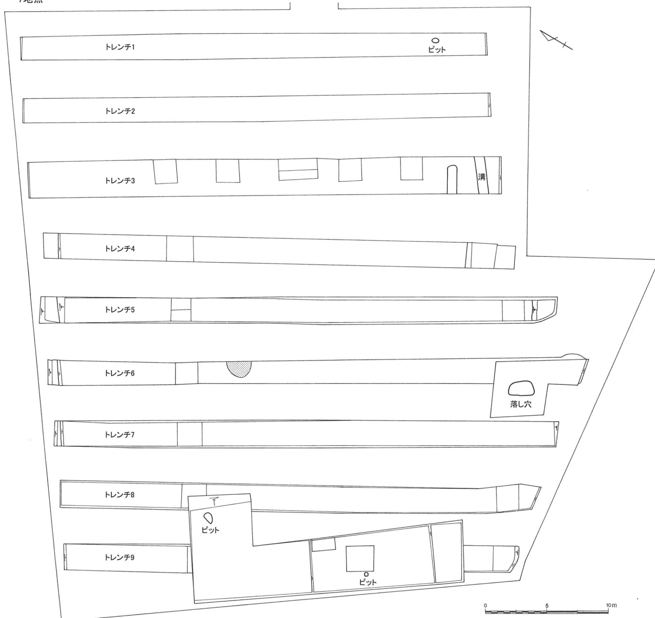
第14図 鶴ヶ舞遺跡第6・7地点調査区域図 (1/300)、土層 (1/150)
