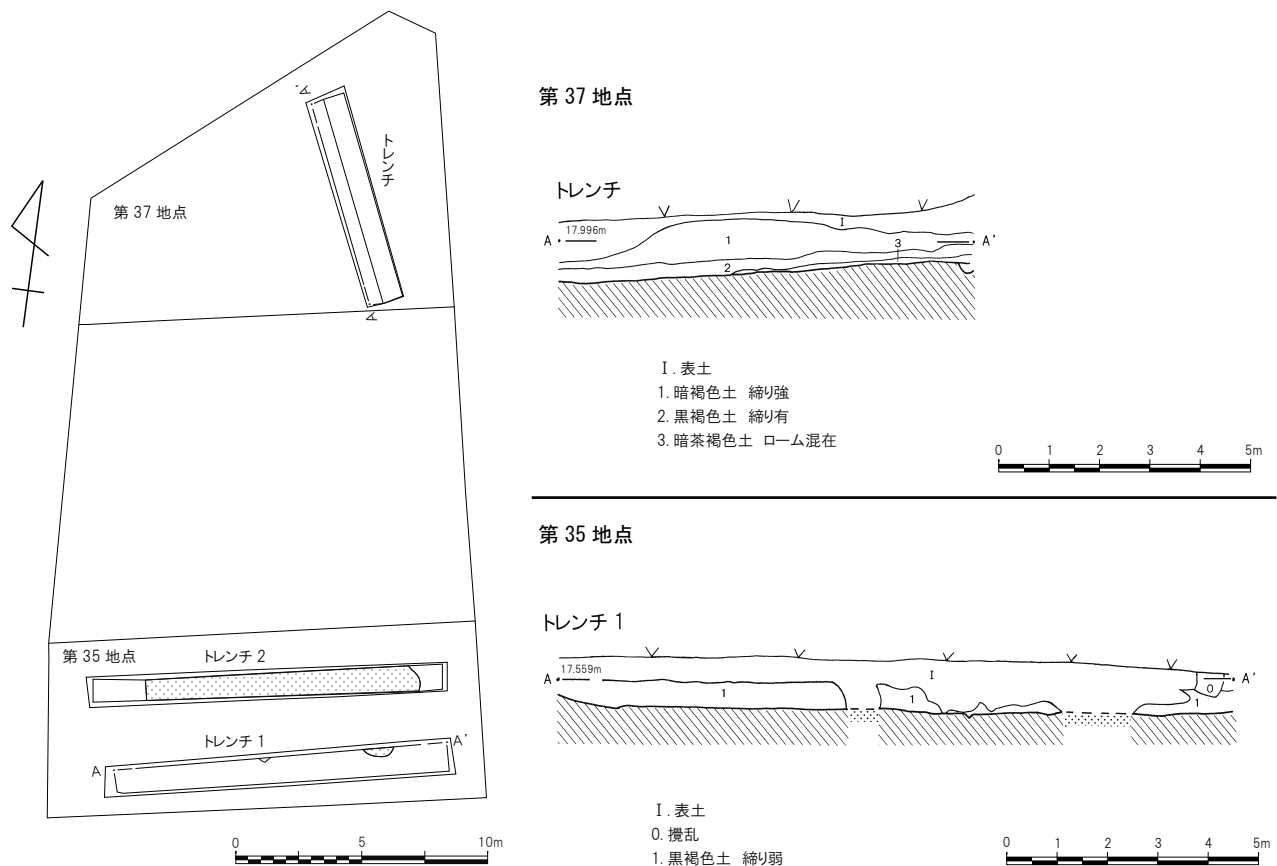
第73図 鶴ヶ舞遺跡第35・37地点調査区域図(1/300)、土層(1/150)
