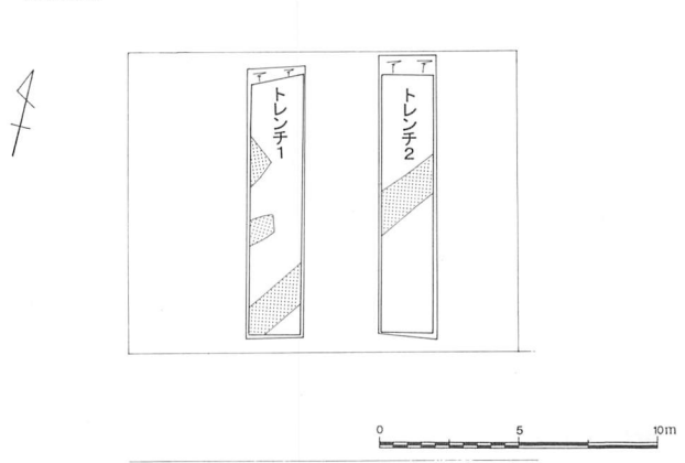
第22図 東久保遺跡第19・20・21・22地点調査区域図 (1/300)・土層 (1/60)
