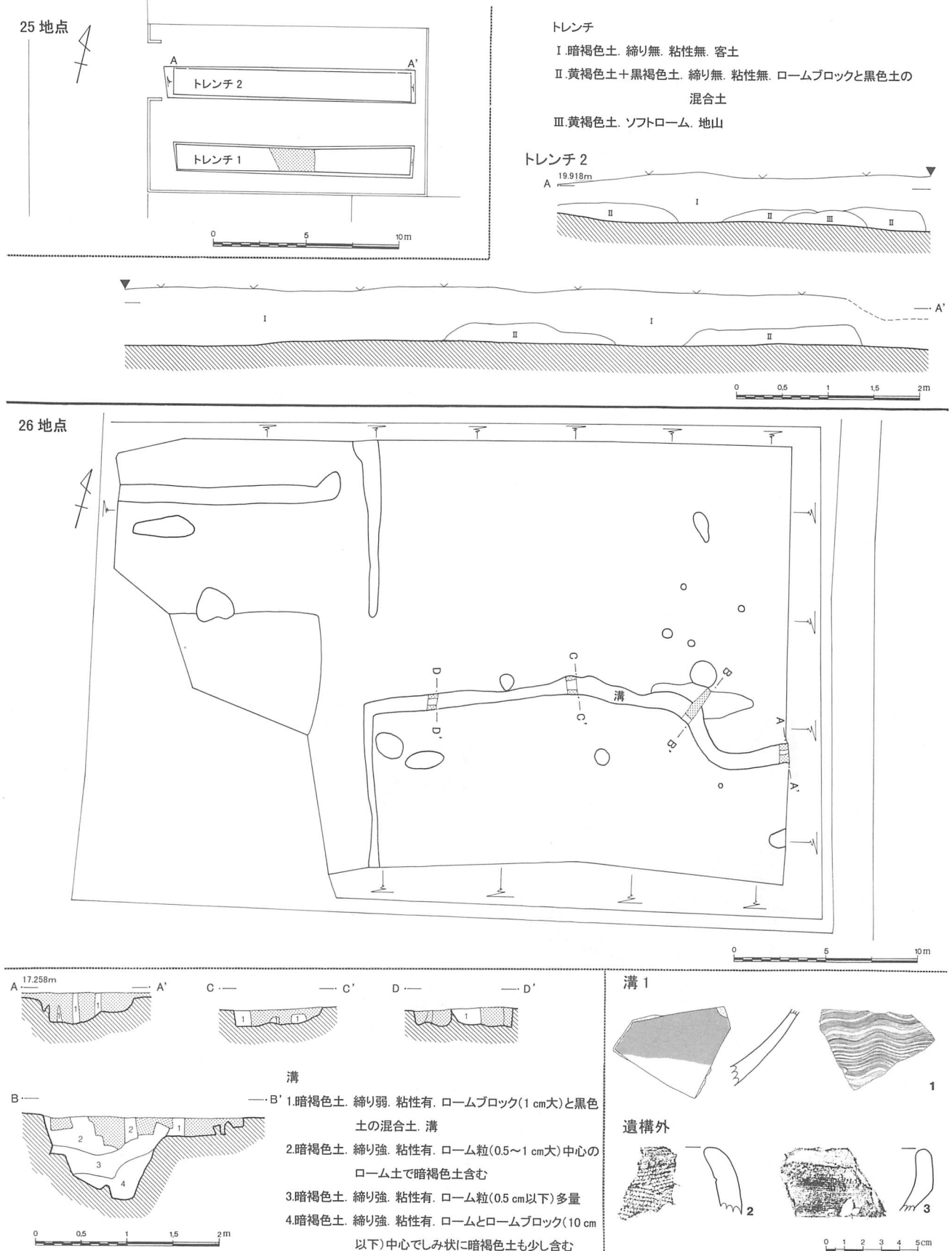
第33図 東久保遺跡第25・26地点遺構配置図(1/300)・土層(1/60)・第26地点出土遺物(1/3)
