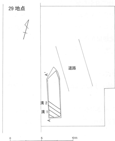
第34図 東久保遺跡第28・29地点遺構配置図(1/300)・土層(1/60)
