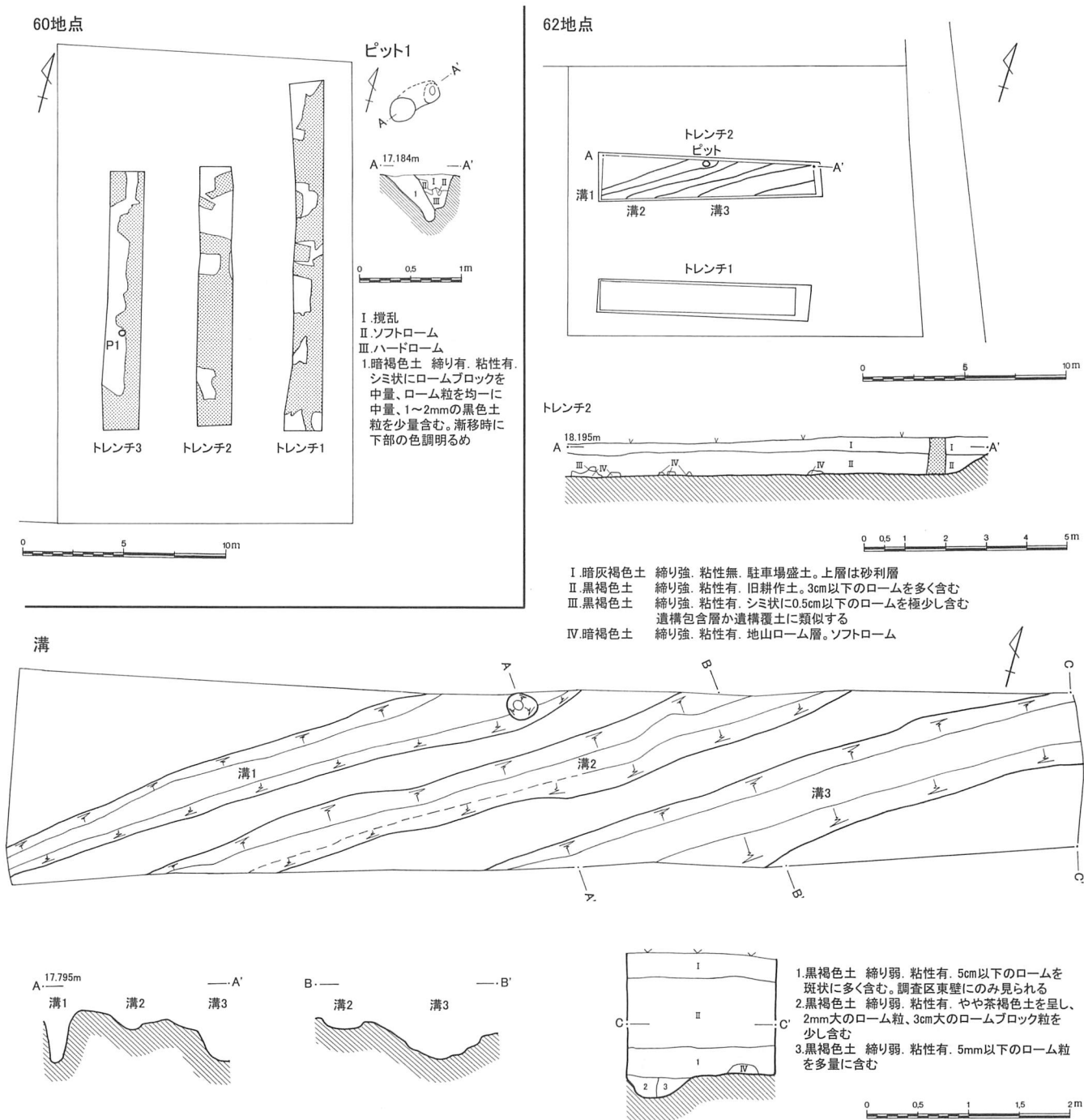
第29図 東久保遺跡第60・62地点遺構配置図 (1/300)、土層 (1/150)、ピット、溝 (1/60)
