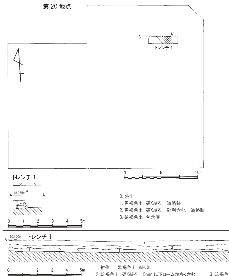
第41図 東久保西遺跡第20地点調査区域図・21地点遺構配置図(1/300)、土層(1/150)、出土遺物(1/4)
