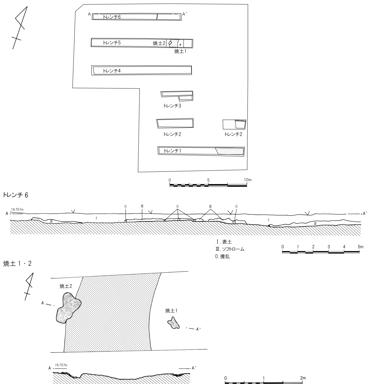
第 99 図 東久保西遺跡第 24 地点遺構配置図 (1/300)、土層 (1/150)、焼土 (1/60)
