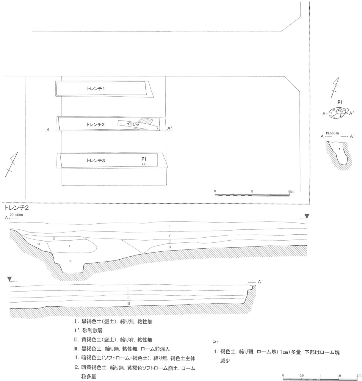
第 28 図 東中学校西遺跡第 13 地点遺構配置図 (1/300)・土層・Pit (1/60)
