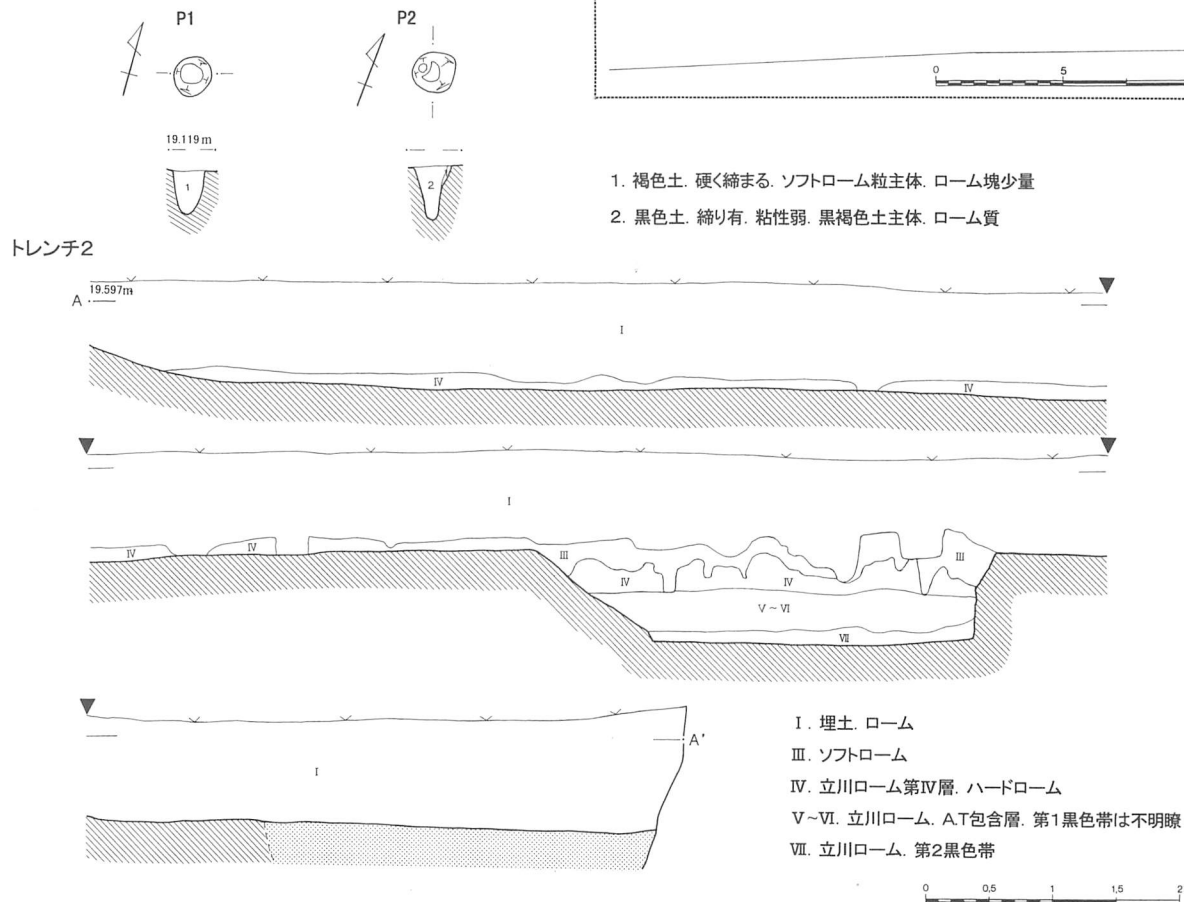
第 32 図 東中学校西遺跡第 16 地点遺構配置図 (1/300)・土層・Pit (1/60)
