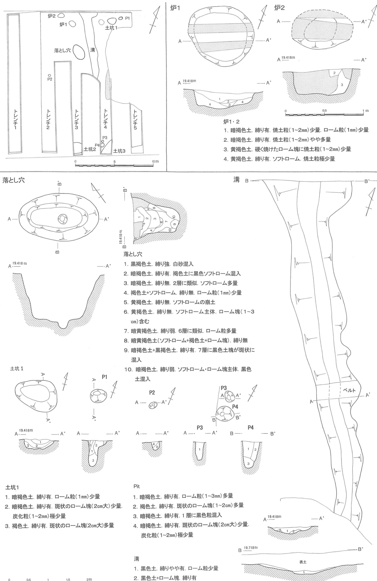
第 37 図 東久保南遺跡第 14 地点遺構配置図 (1/300)・炉 (1/30)・落とし穴・土坑・Pit・溝 (1/60)
