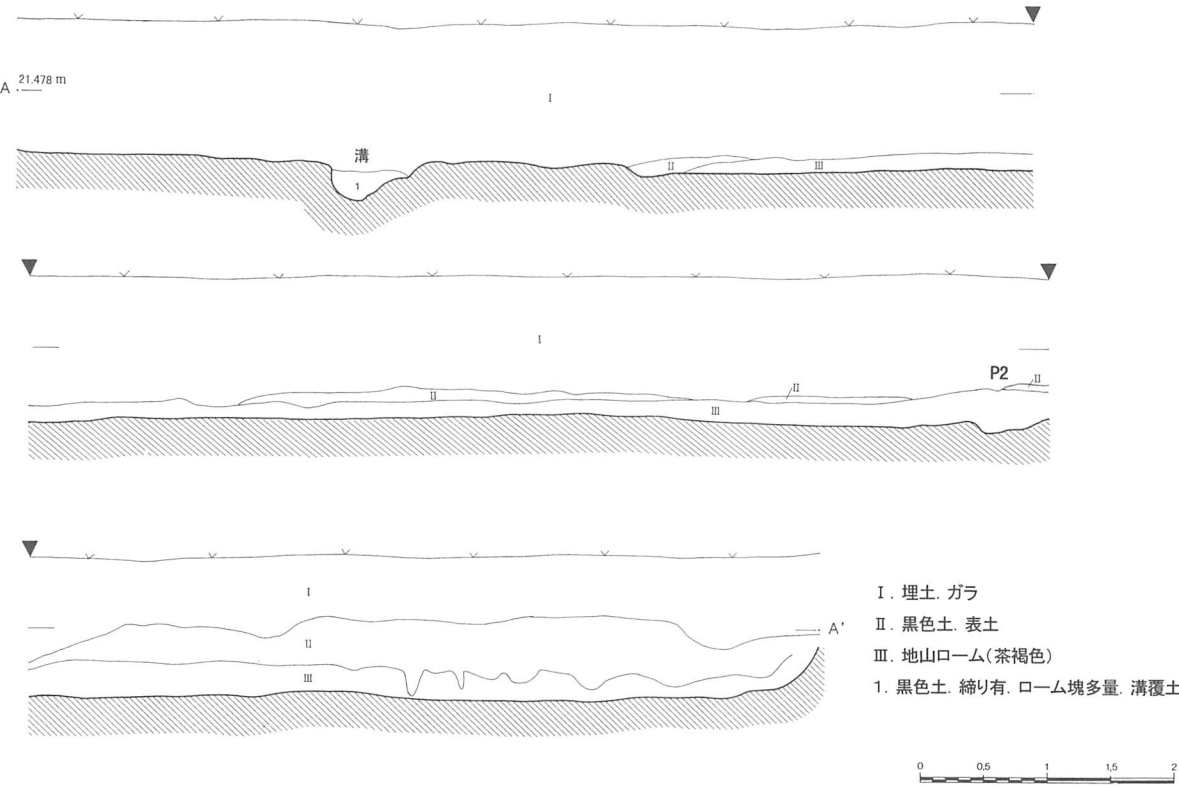
第 40 図 東久保南遺跡第 17 地点遺構配置図 (1/300)・土層 (1/60)
