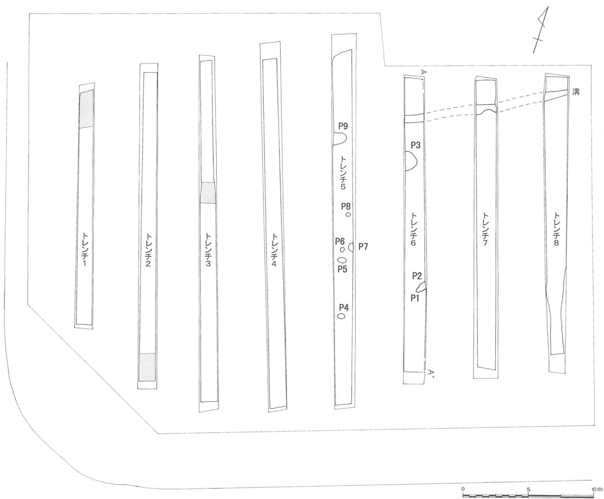
トレンチ6
