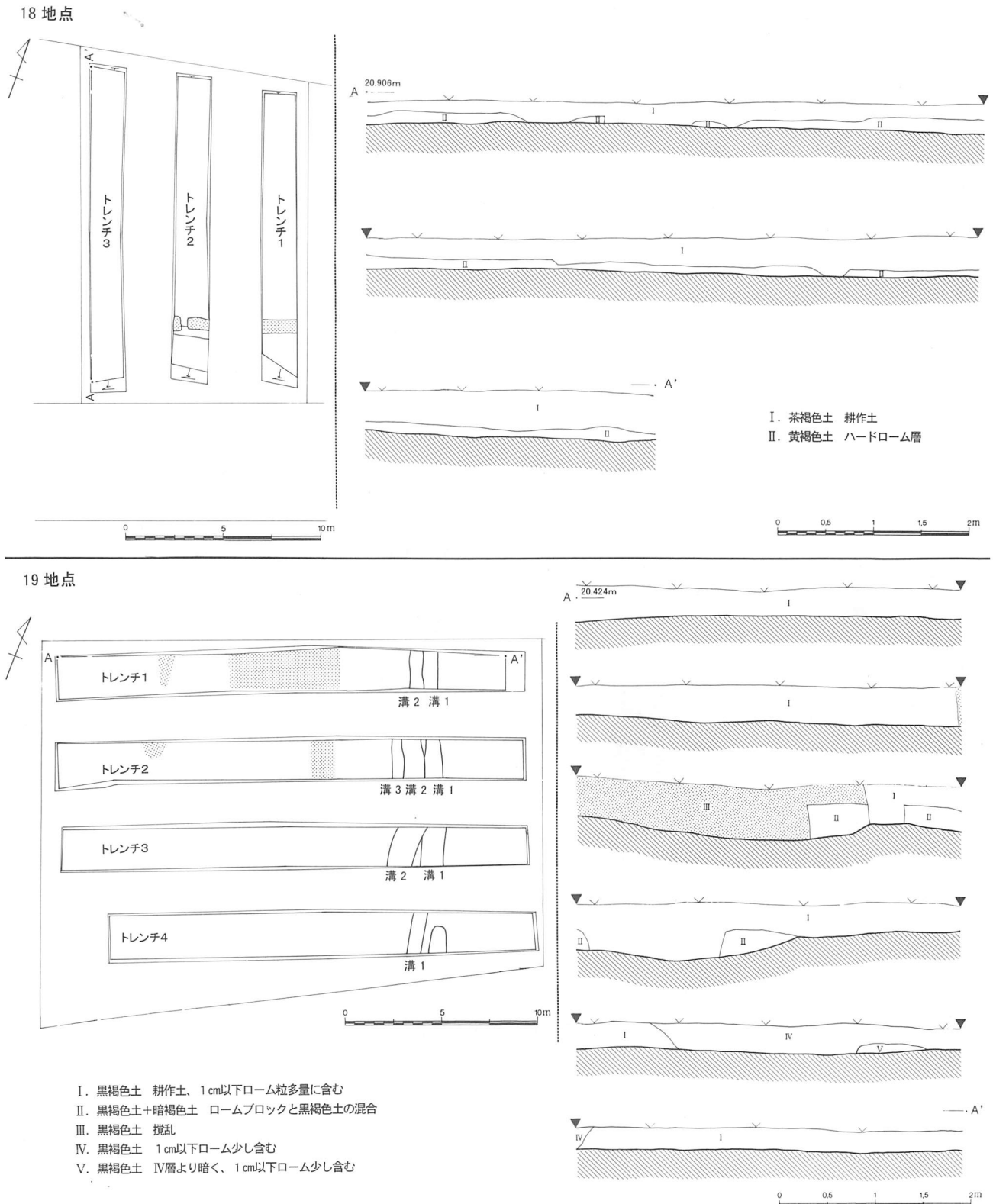
第35図 東久保南遺跡第18・19地点調査区域図 (1/300)・土層 (1/60)
