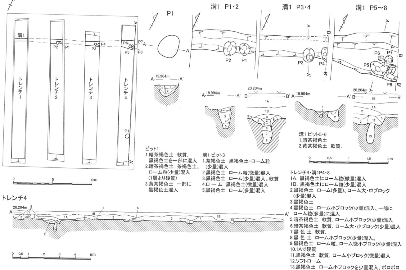
第37図 東久保南遺跡第27・28地点遺構配置図 (1/300)、土層 (1/150)、溝、ピット (1/60)
