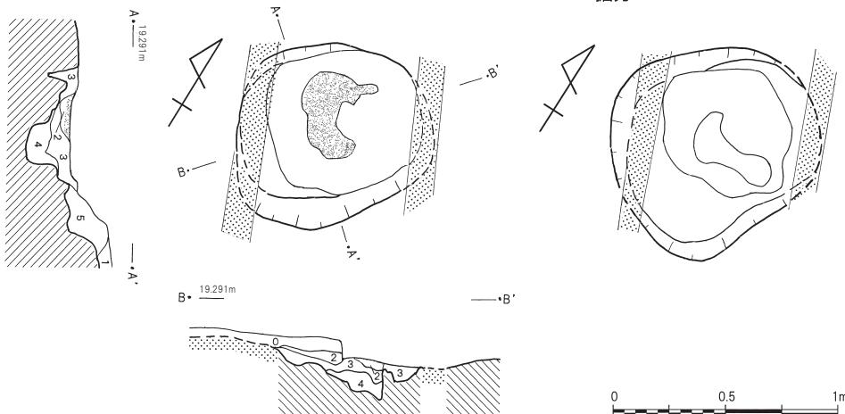
第34図 東久保南遺跡第43地点 J3号住居跡・遺物出土状況 (1/60)、炉・掘方 (1/30)
