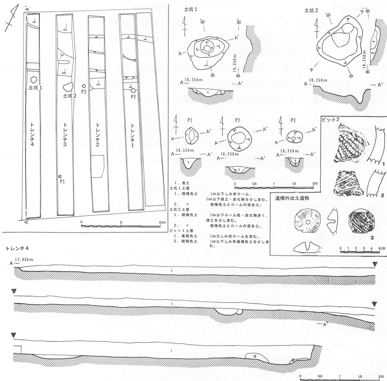
第44図 西ノ原遺跡第100地点遺構配置図 (1/300)・土坑・ピット・土層 (1/60)・出土遺物 (1/3)
