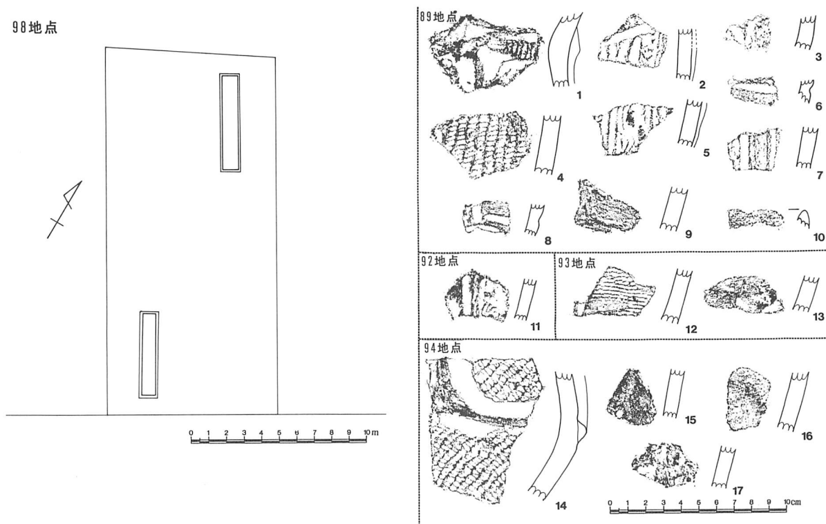
第56図 西ノ原遺跡第98地点調査区域図(1/300)・第89・91・93・94地点出土遺物(1/3)
