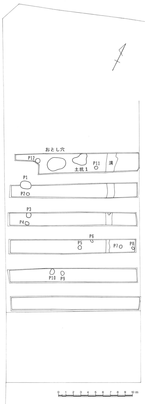
第52図 西ノ原遺跡第99地点遺構配置図(1/300)
