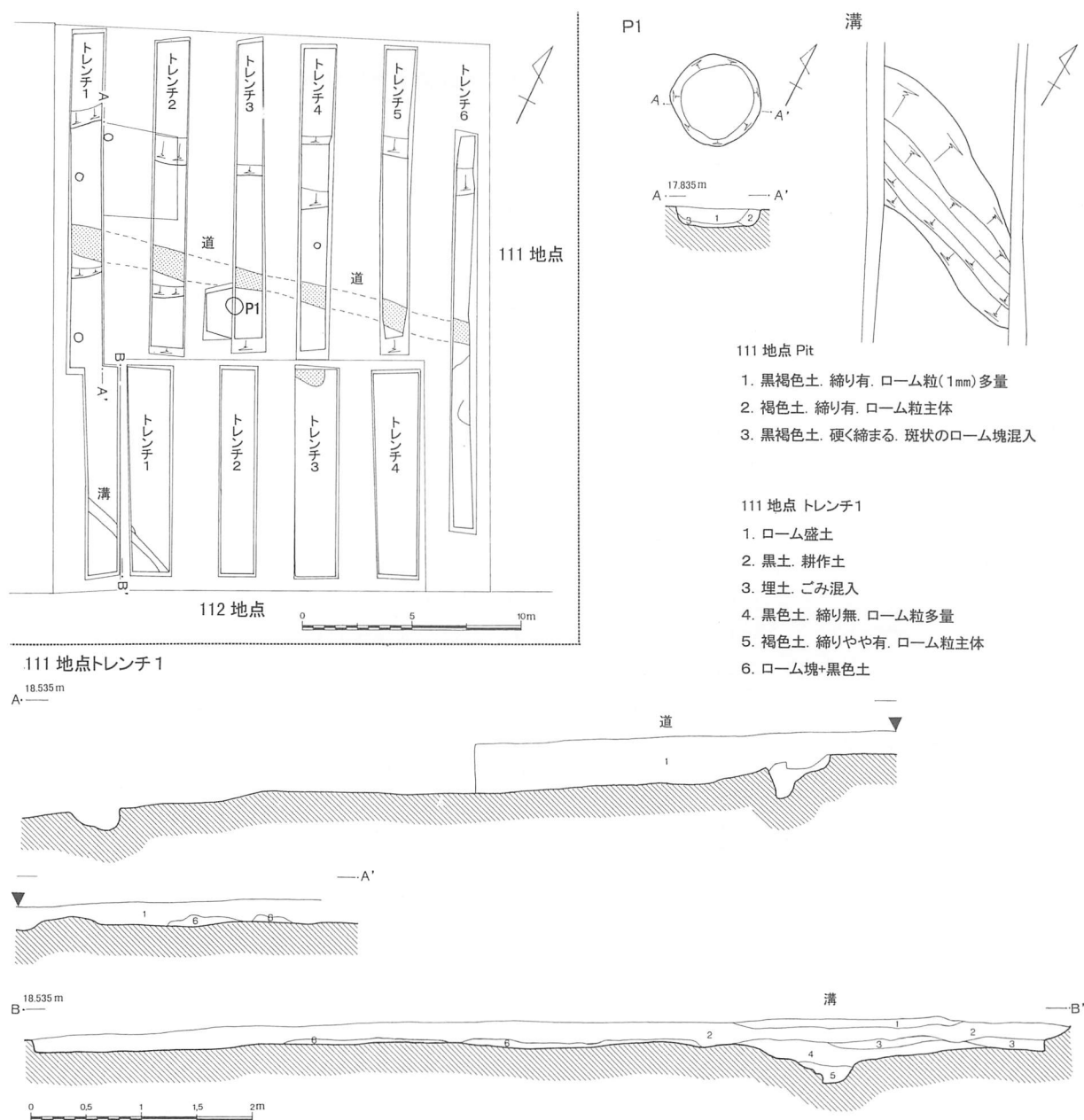
第45図 西ノ原遺跡第111・112地点遺構配置図(1/300)・土層・Pit・溝(1/60)
