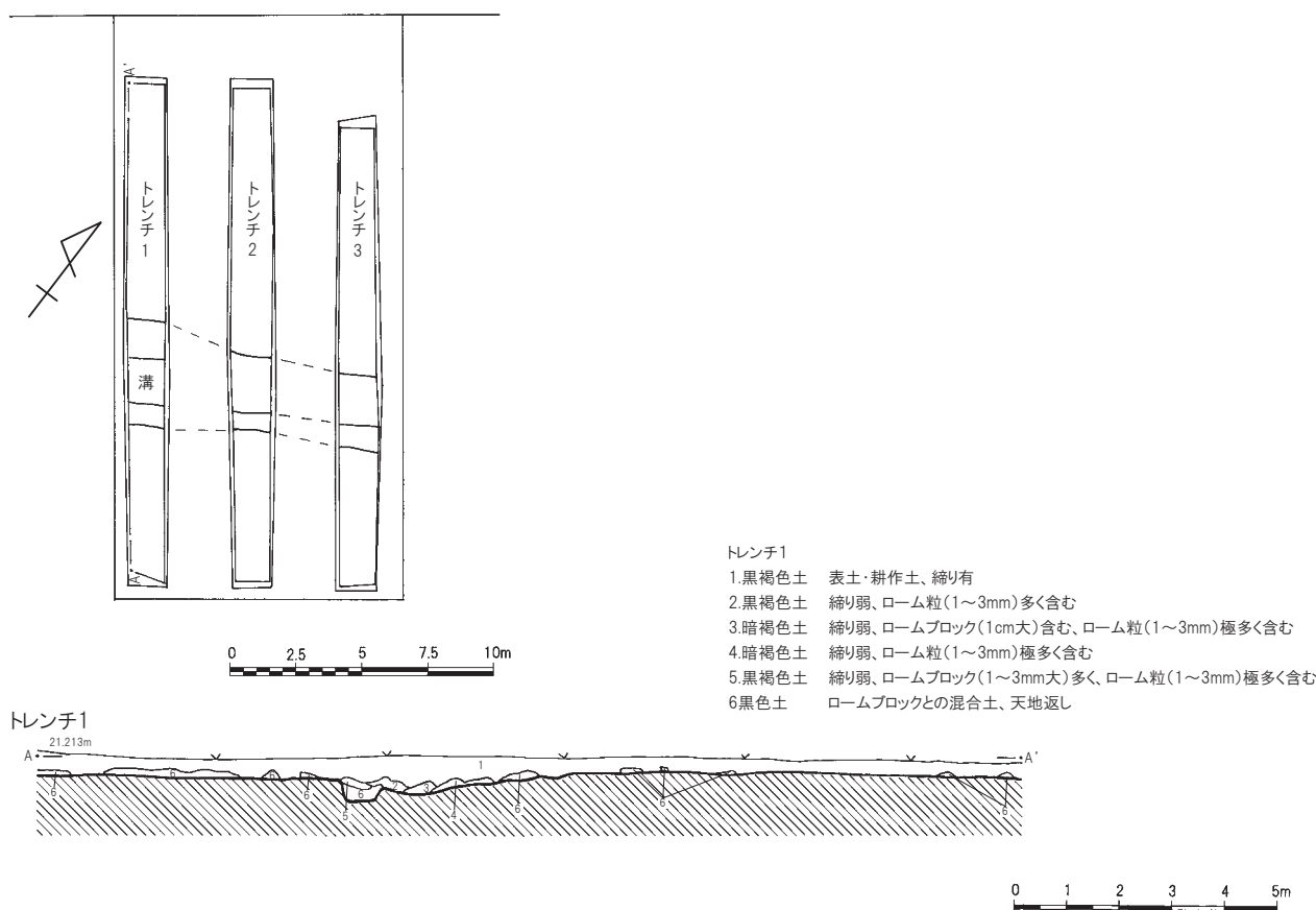
第53図 西ノ原遺跡第146地点 遺構配置図(1/300)、土層図(1/150)
