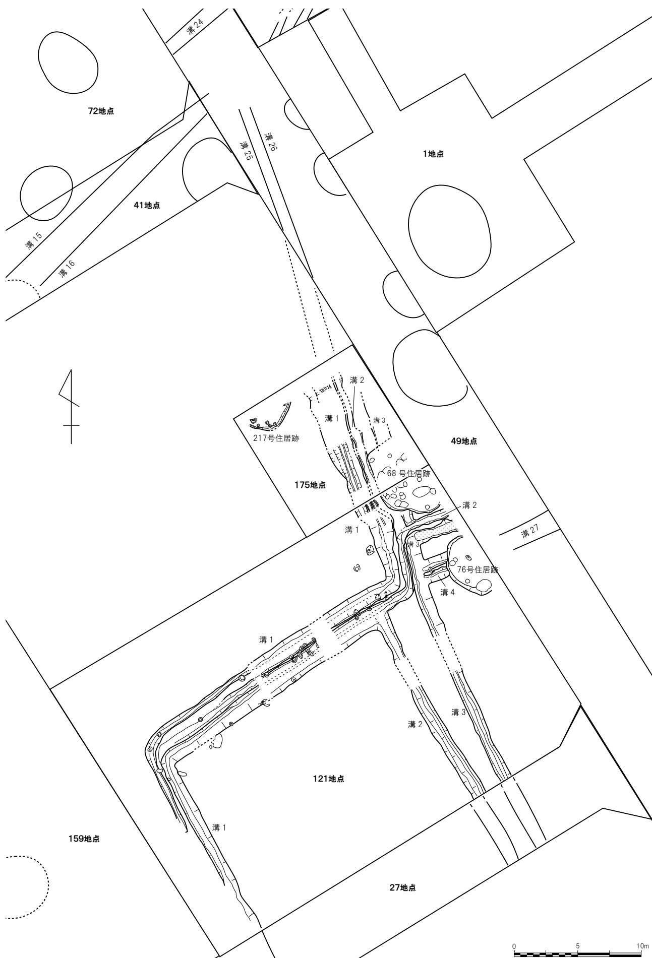
第 119 図 西ノ原遺跡第 175 地点溝配置図 (1/300)
