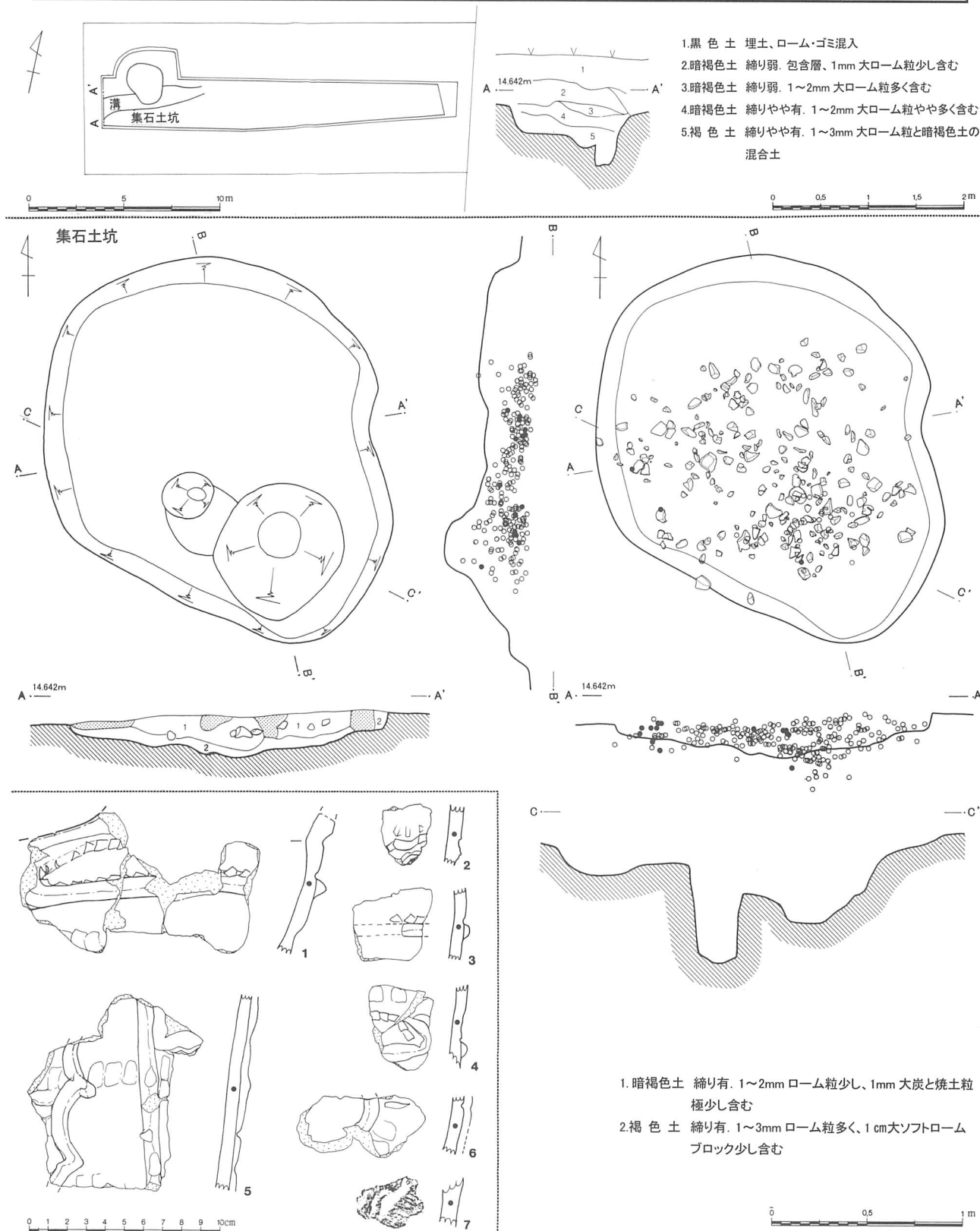
第57図 神明後遺跡第15地点遺構配置図（1/300）、集石土坑（1/30）、出土土器（1/3）
