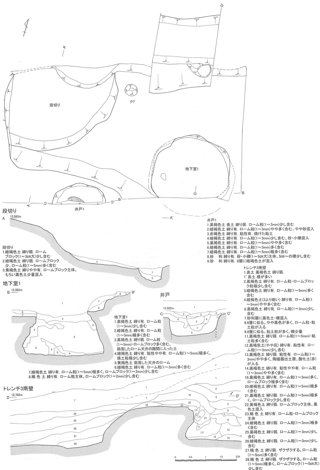
第65図 神明後遺跡第21地点地下室1、井戸、段切り状遺構(1/60)
