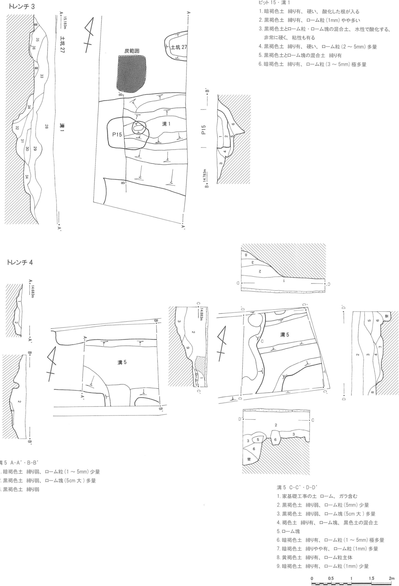
第 104 図 神明後遺跡第 33 地点トレンチ 3・4 溝・土坑・ピット (1/60)
