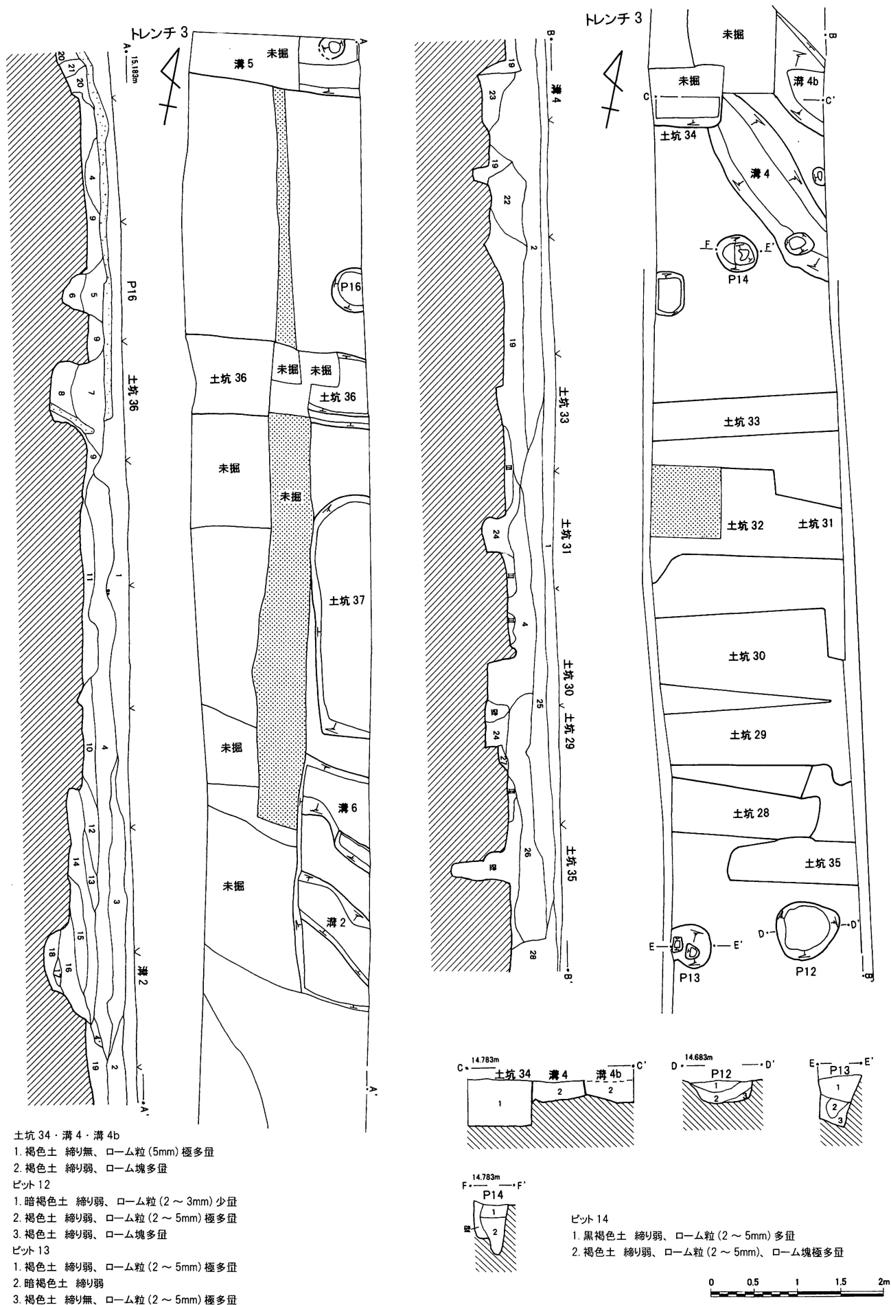
第 103 図 神明後遺跡第 33 地点トレンチ 3 溝・土坑・ピット (1/60)
