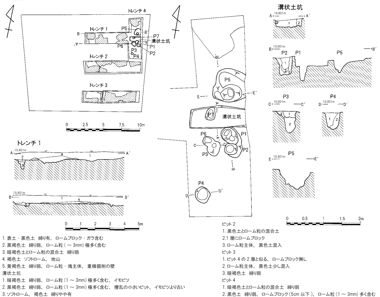
第 69 図 神明後遺跡第 42・43 地点遺構配置図 (1/300)、土層図 (1/150)、溝状土坑・ピット (1/60)
