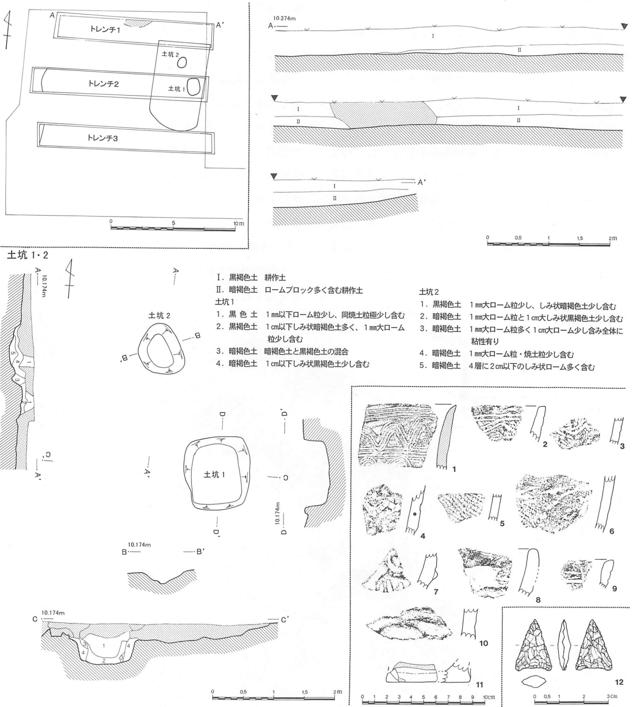
第51図 苗間東久保遺跡第21地点遺構配置図 (1/300) ・土層・土坑 (1/60) ・出土遺物 (1/3) (2/3)
