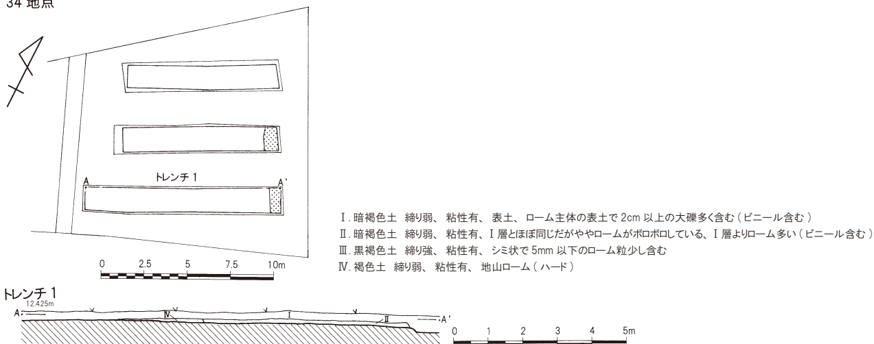
第81図 浄禅寺跡遺跡第25・34地点調査区域図(1/300)、土層(1/150)
