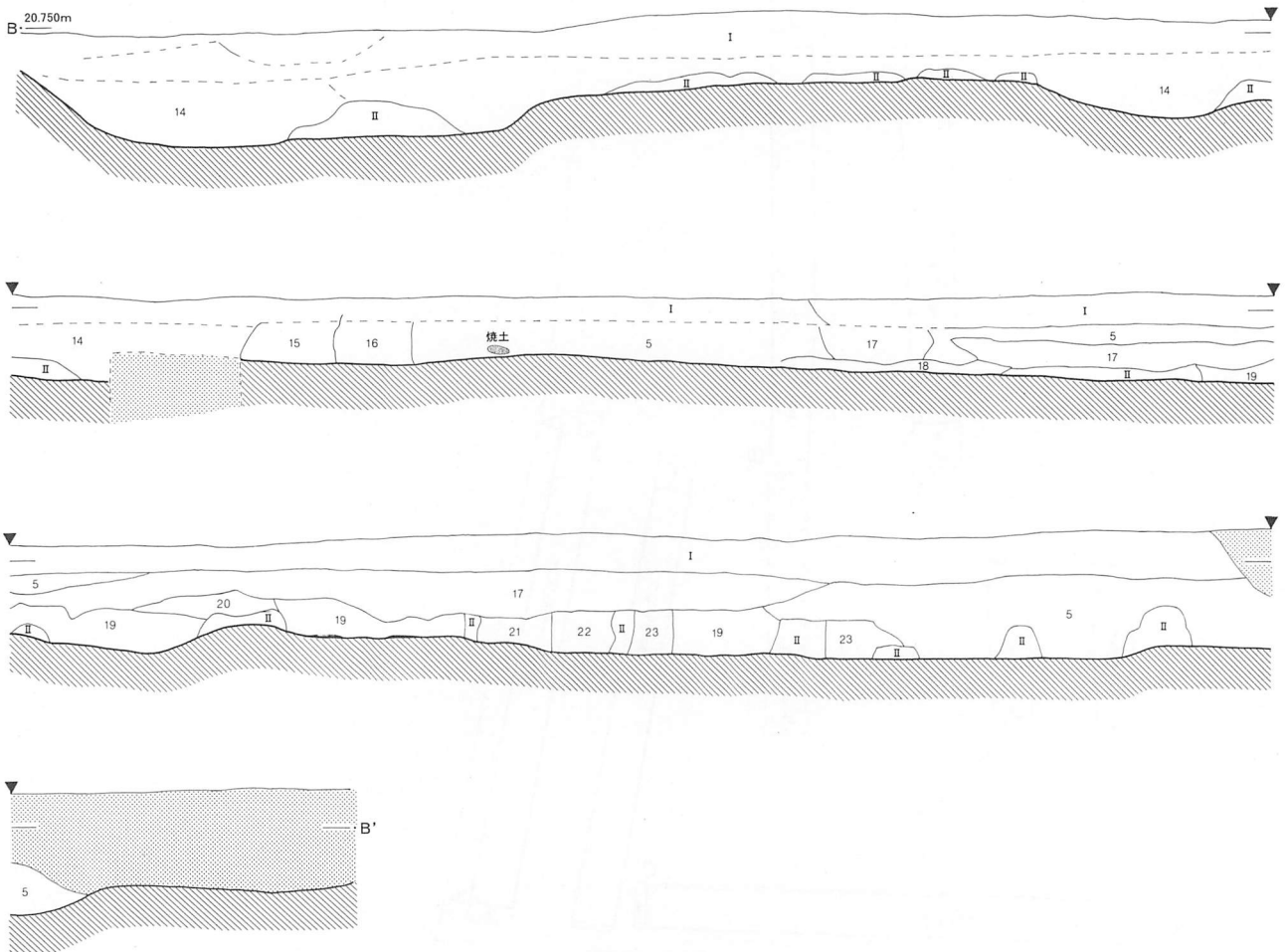
第73図 大井宿遺跡第5地点土層 (1/60)
