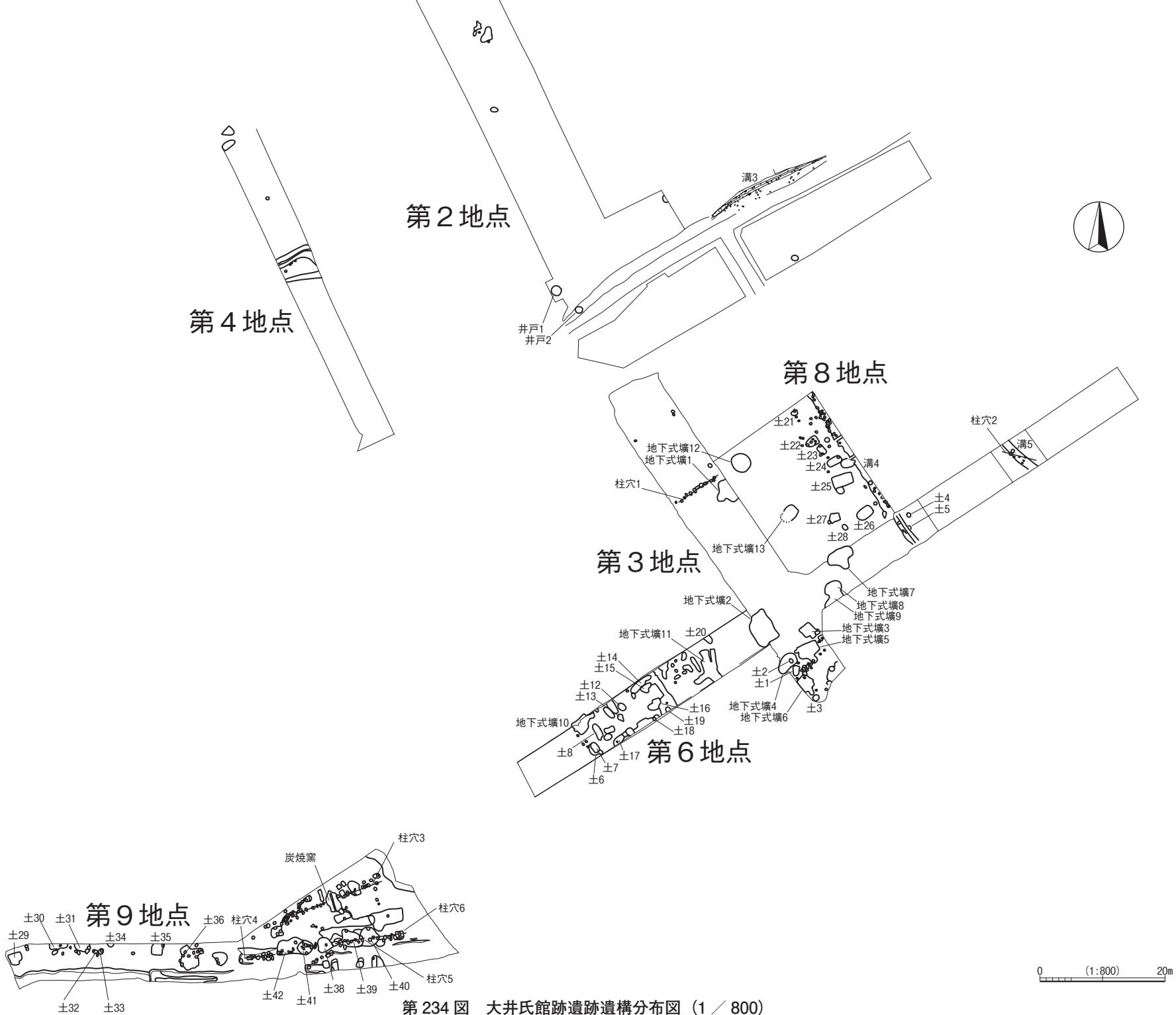
第 234 図 大井氏館跡遺跡遺構分布図 (1 / 800)
