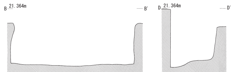
第 238 図 大井氏館跡遺跡 地下式墳 2 (1 / 80)
