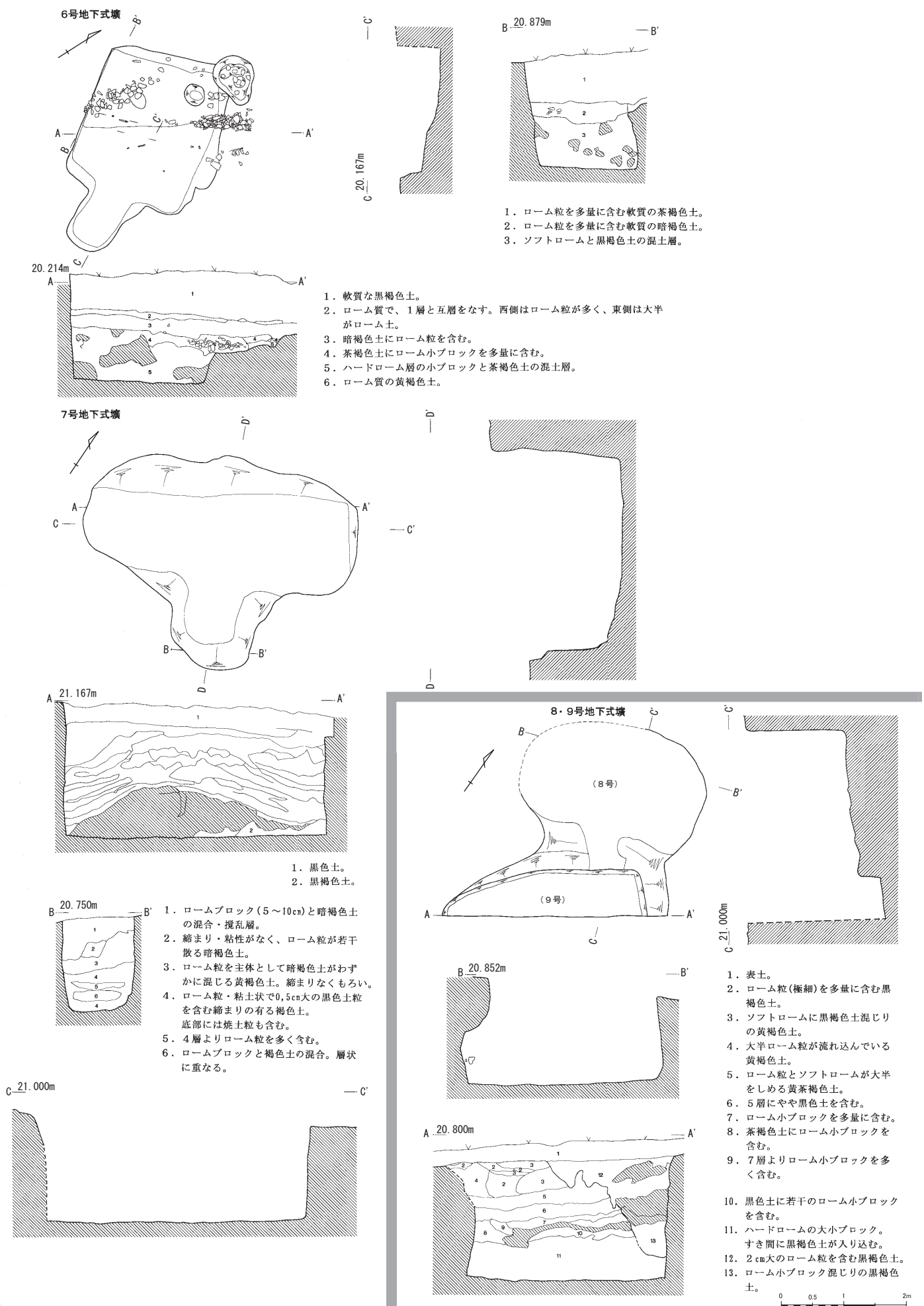
第240図 大井氏館跡遺跡 地下式墳4 (1/80)
