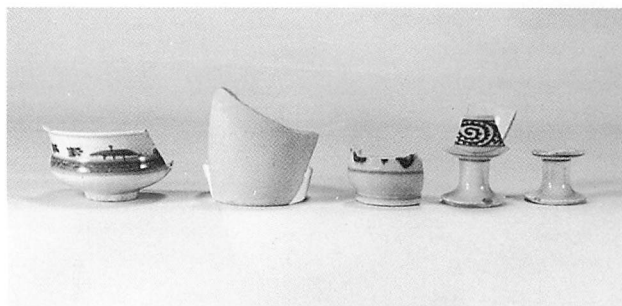
磁器 (No.23~27)
