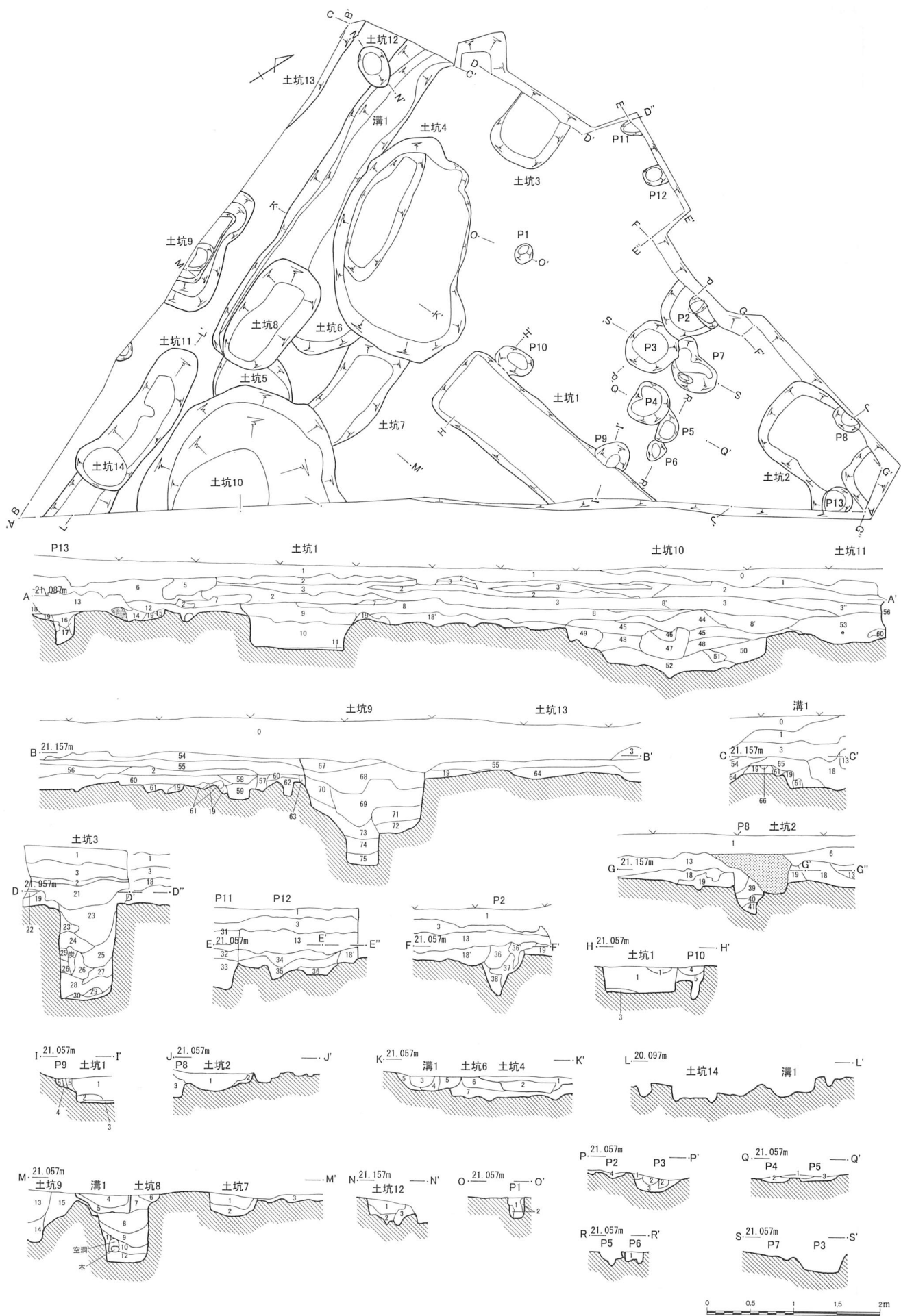
第91図 大井氏館跡遺跡第17地点土坑、溝、ピット (1/60)
