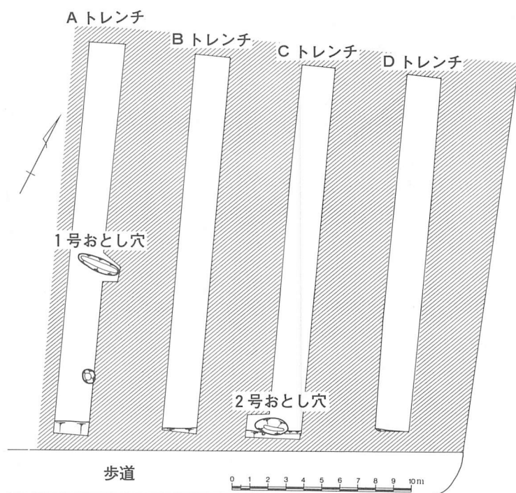
第55図 本村遺跡第10地点遺構配置図 ( \frac{1}{300} )
