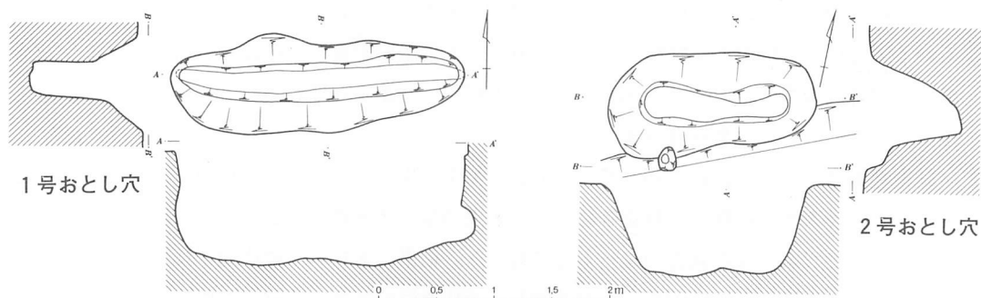
第56図 本村遺跡第10地点おとし穴 ( \frac{1}{60} )
