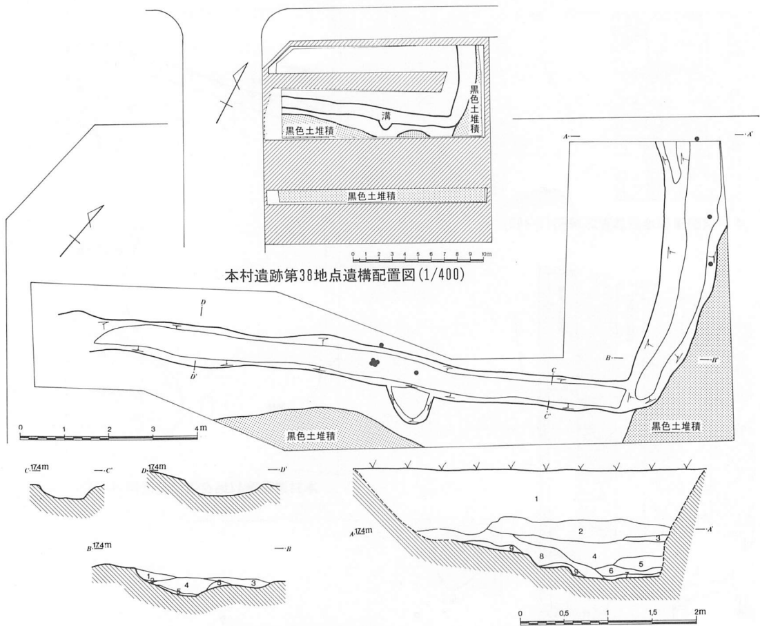
本村遺跡第38地点溝 平面図(1/120)・断面図(1/60)
