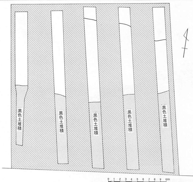
本村遺跡第38地点溝 平面図(1/120)・断面図(1/60)
