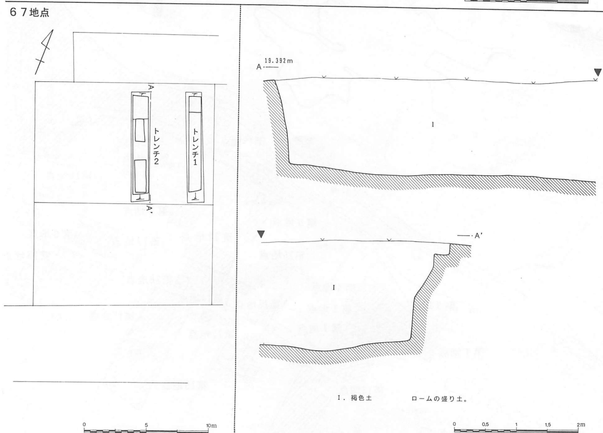
第87図 本村遺跡第66・67地点遺構配置図(1/300)・ 土層(1/60)
