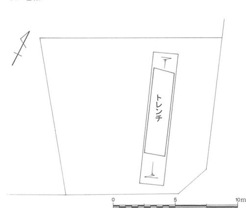
第95図 本村遺跡第80地点遺構配置図 (1/300)・土坑・ピット (1/60)・第81・82・83地点調査区域図 (1/300)
