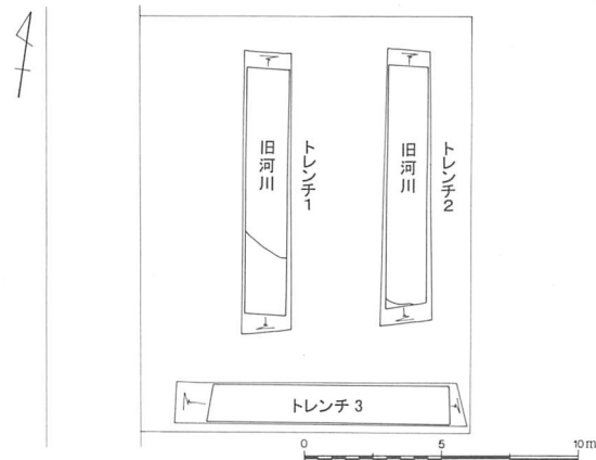
第95図 本村遺跡第80地点遺構配置図 (1/300)・土坑・ピット (1/60)・第81・82・83地点調査区域図 (1/300)
