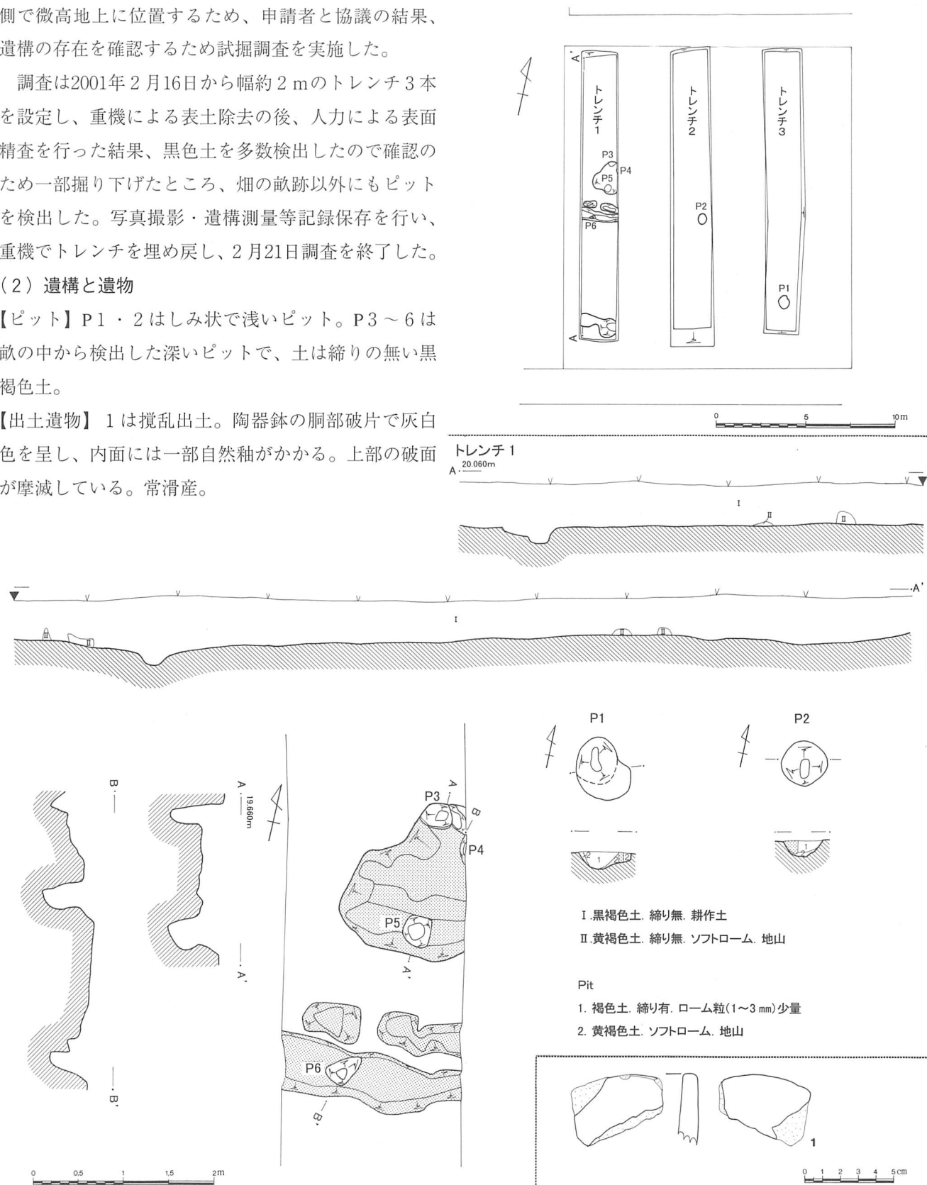
第92図 本村遺跡第93地点遺構配置図(1/300)・土層・ピット(1/60)・出土遺物(1/3)
